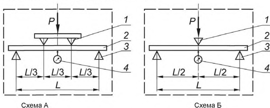
1 — призмы для передачи изгибающего усилия; 2 — образец; 3 — опорные призмы, 4 — индикатор, P — нагрузка
