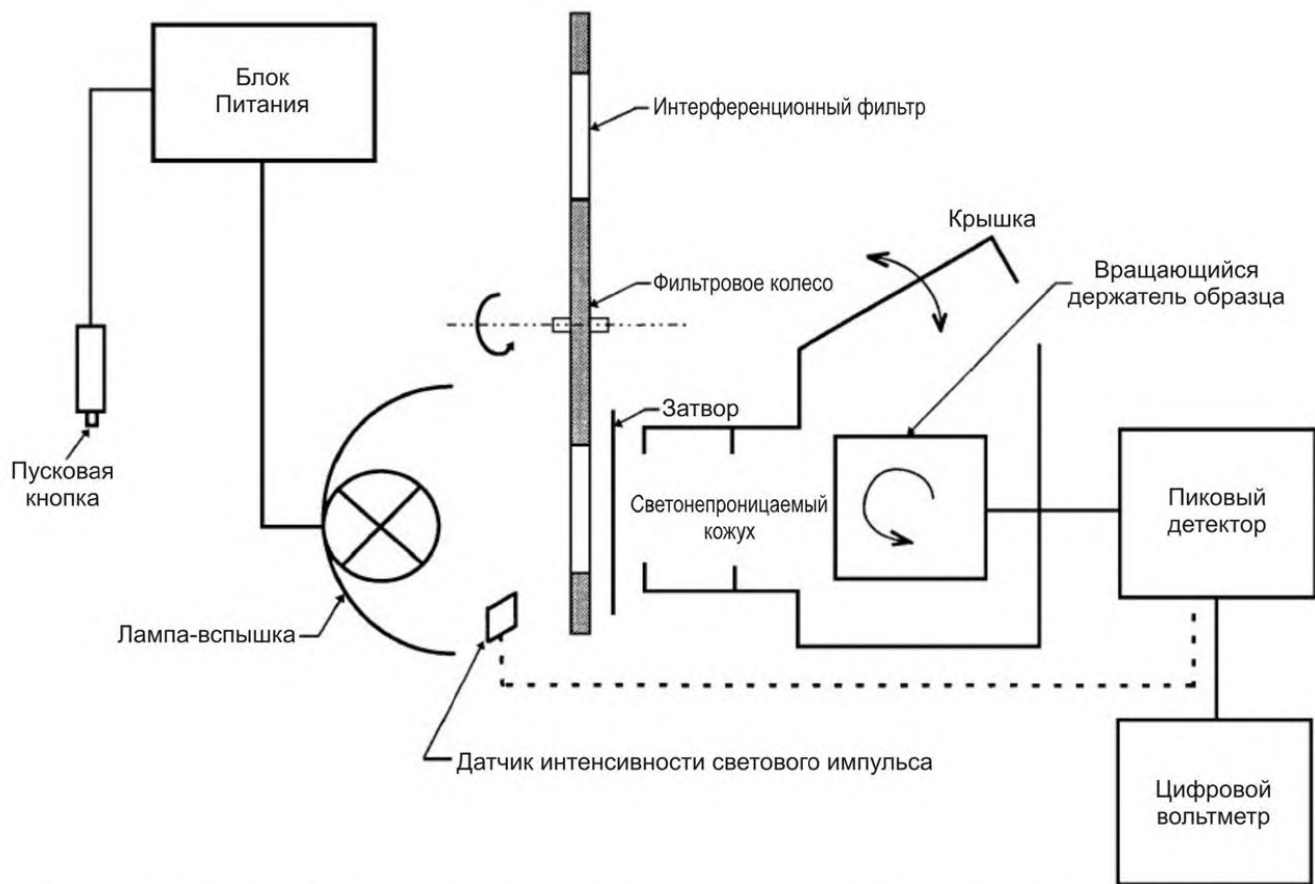
Рисунок А.3 Установка для измерения спектральной чувствительности при использовании импульсного излучения
