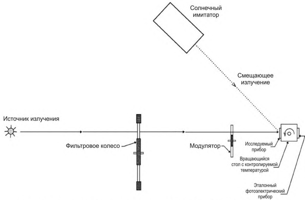
Рисунок А.2 Измерения спектральной чувствительности с помощью фильтрового колеса
