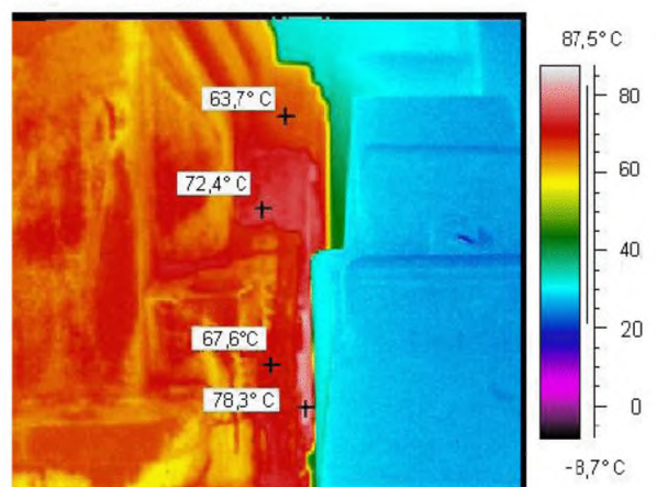
Рисунок С.4 – Редуктор со стороны входного вала
