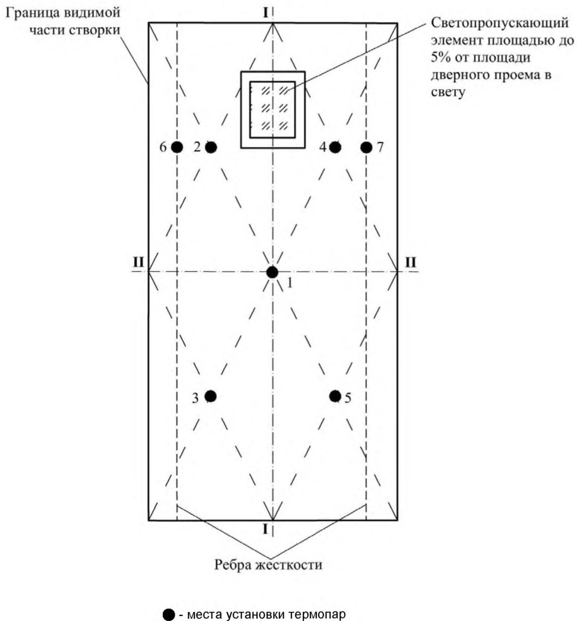
Рисунок А.1 - Схема установки термопар на необогреваемой поверхности створок одностворчатой распашной и сплошной горизонтально-раздвижной двери бокового открывания и со светопронускающим элементом створок до 5% от площади дверного проема в свету
