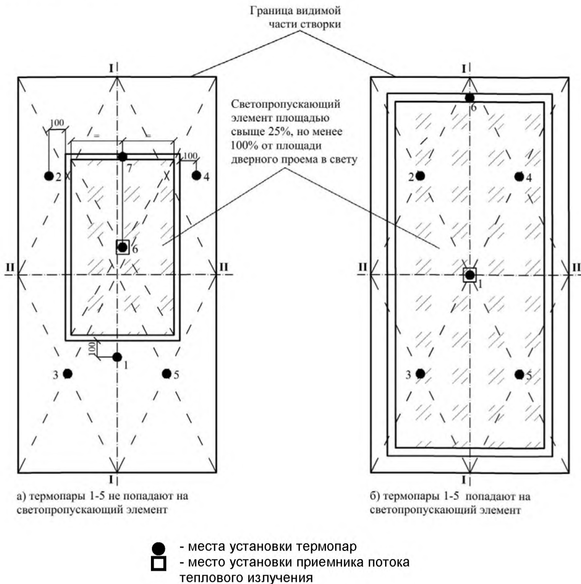
Рисунок А.3 - Схема установки термопар и приемника потока теплового излучения на необогреваемой поверхности створки одностворчатой распашной и горизонтально-раздвижной двери бокового открывания со светопроницающим элементом створки свыше 25% но менее 100% от площади проема в свету
