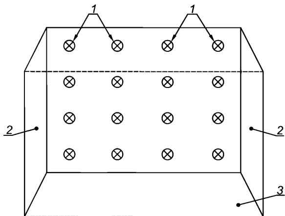
1 – лампы; 2 – алюминиевая фольга; 3 – плоскость образцов Рисунок С.1 – б) Расположение образцов для испытания облучением
