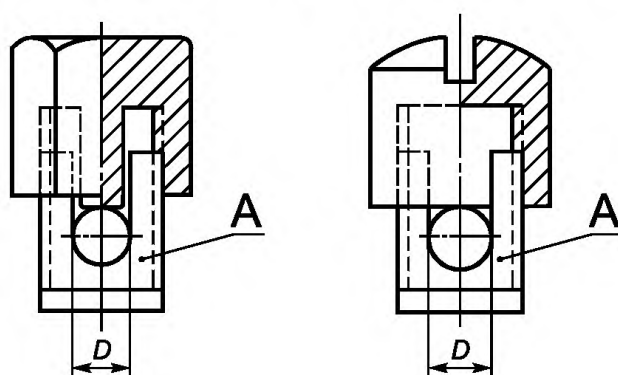
Рисунок 4 — Примеры зажимов под наконечник
