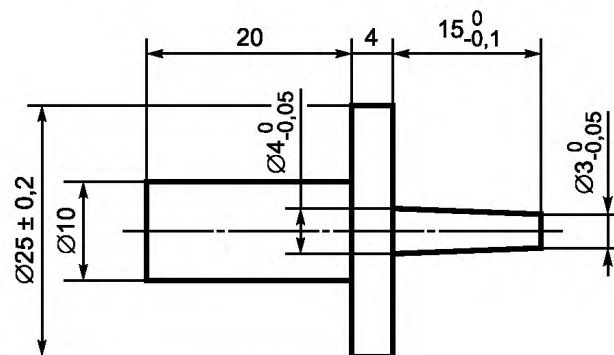
Рисунок 13 — Испытательный стержень
