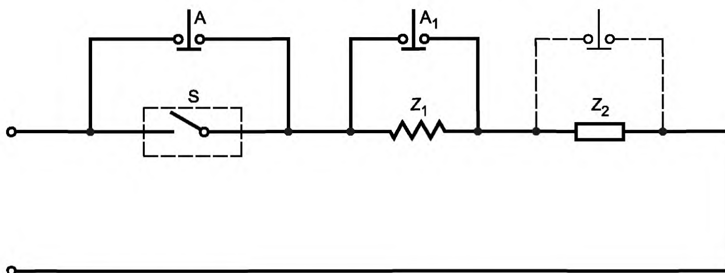
Рисунок 18 — Схема для испытания на нагрев
