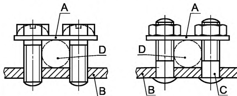
Рисунок 2 — Примеры винтовых и шпилечных зажимов
