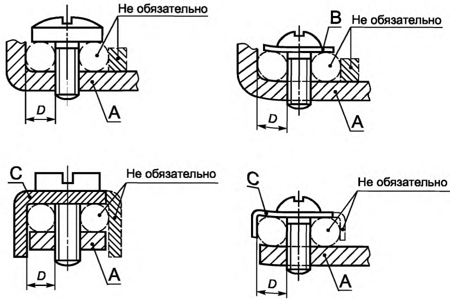
Рисунок 2а — Винтовые зажимы
