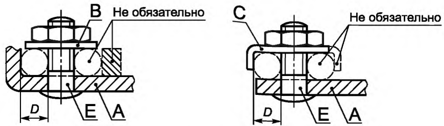
Рисунок 2б — Шпилечные зажимы
