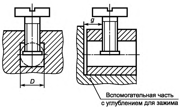
Рисунок 1b — Примеры колонковых зажимов с прижимными пластинами
