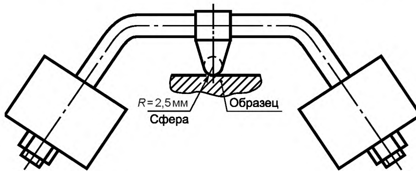
Рисунок 12 — Устройство для вдавления шарика
