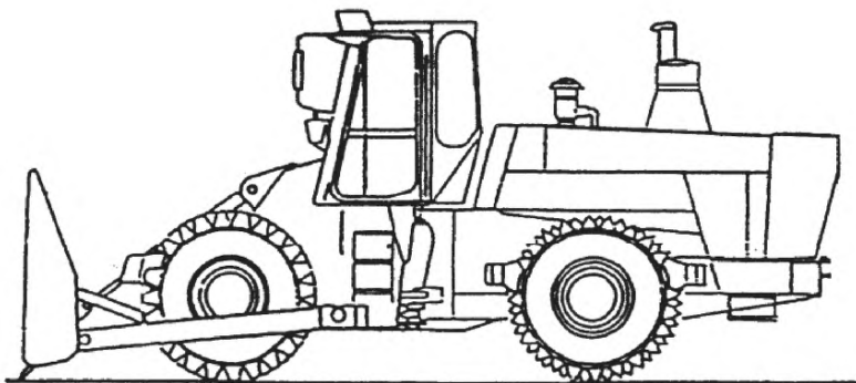
Рисунок В.2 – Уплотняющая машина с бульдозерным оборудованием
