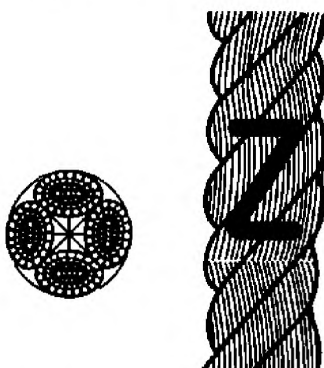
Рисунок 2 – Конфигурация 4-рядного (shroud-laid) каната (тип В)
