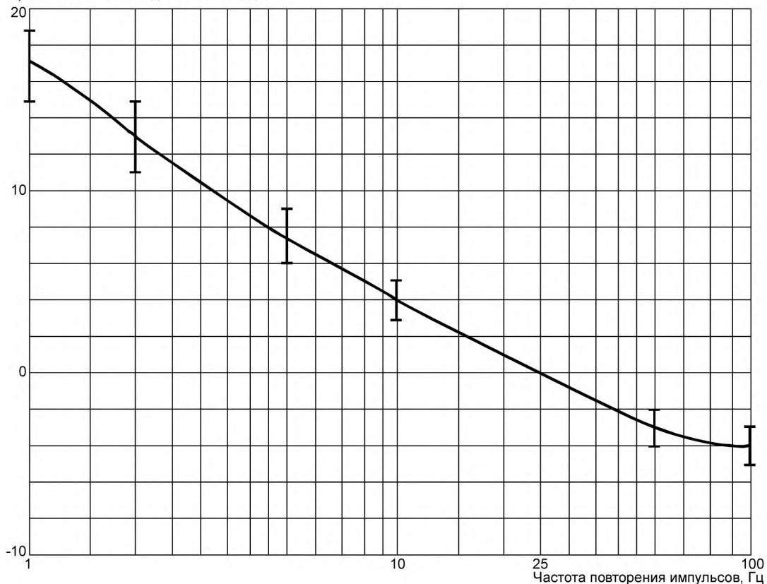
а) Импульсная характеристика ИП для полосы частот А (от 9 до 150 кГц) и допускаемые отклонения ее значений
