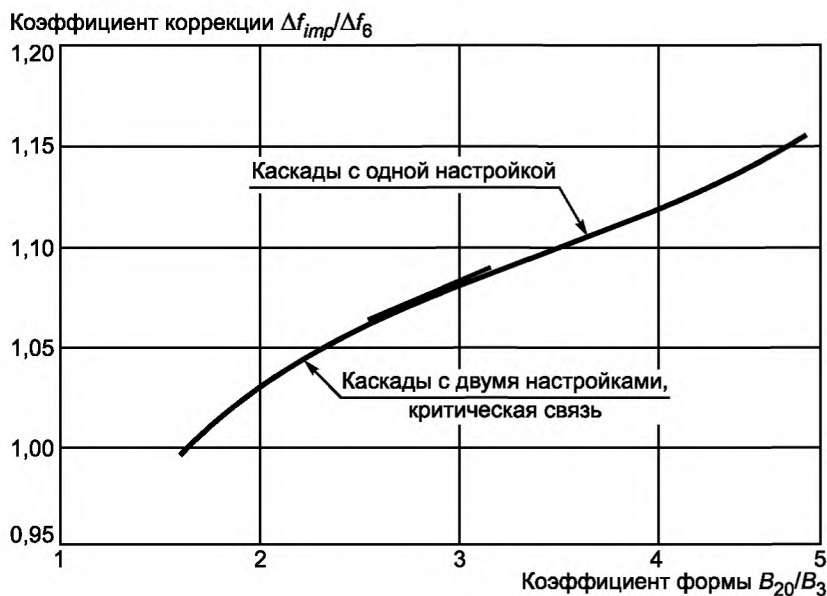
Рисунок Е.1 — Коэффициент коррекции для оценки отношения B_{imp}/B_6 для других типов настраиваемых схем
