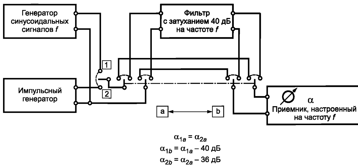
Рисунок 3 – Схема измерения ослабления продуктов интермодуляции
