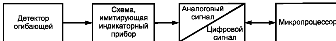
Рисунок 4 — Блок-схема детектора средних значений
