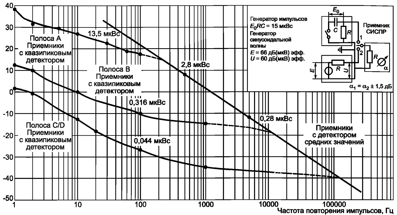
d) Теоретические кривые импульсной характеристики ИП с квазипиковым детектором и детектором средних значений (см. 6.4.2)
