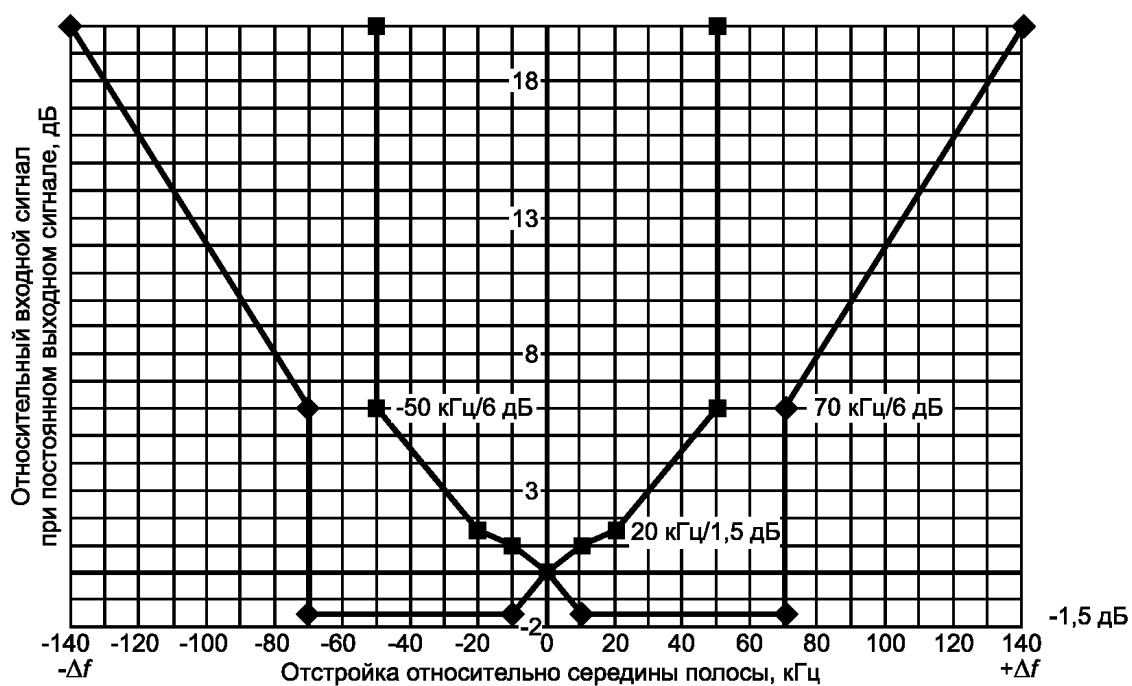
с) Пределы характеристики частотной избирательности ИП для полос частот С и D (от 30 до 1000 МГц)
