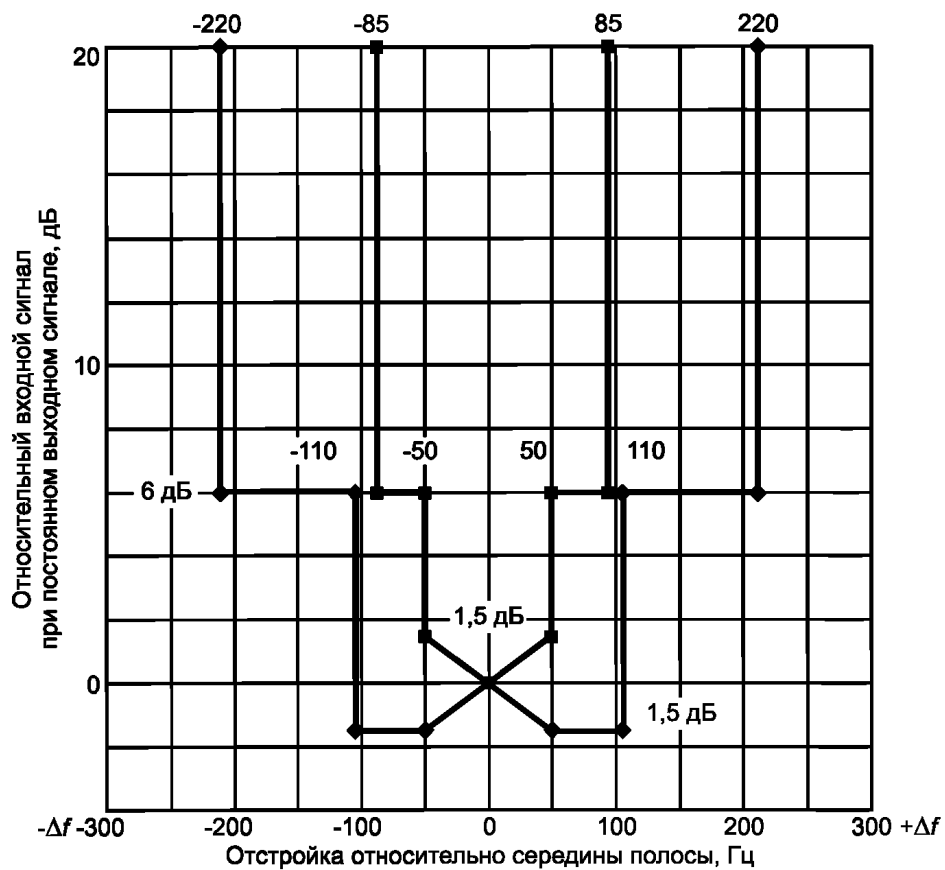
a) Пределы характеристики частотной избирательности ИП для полосы частот А (от 9 до 150 кГц)
