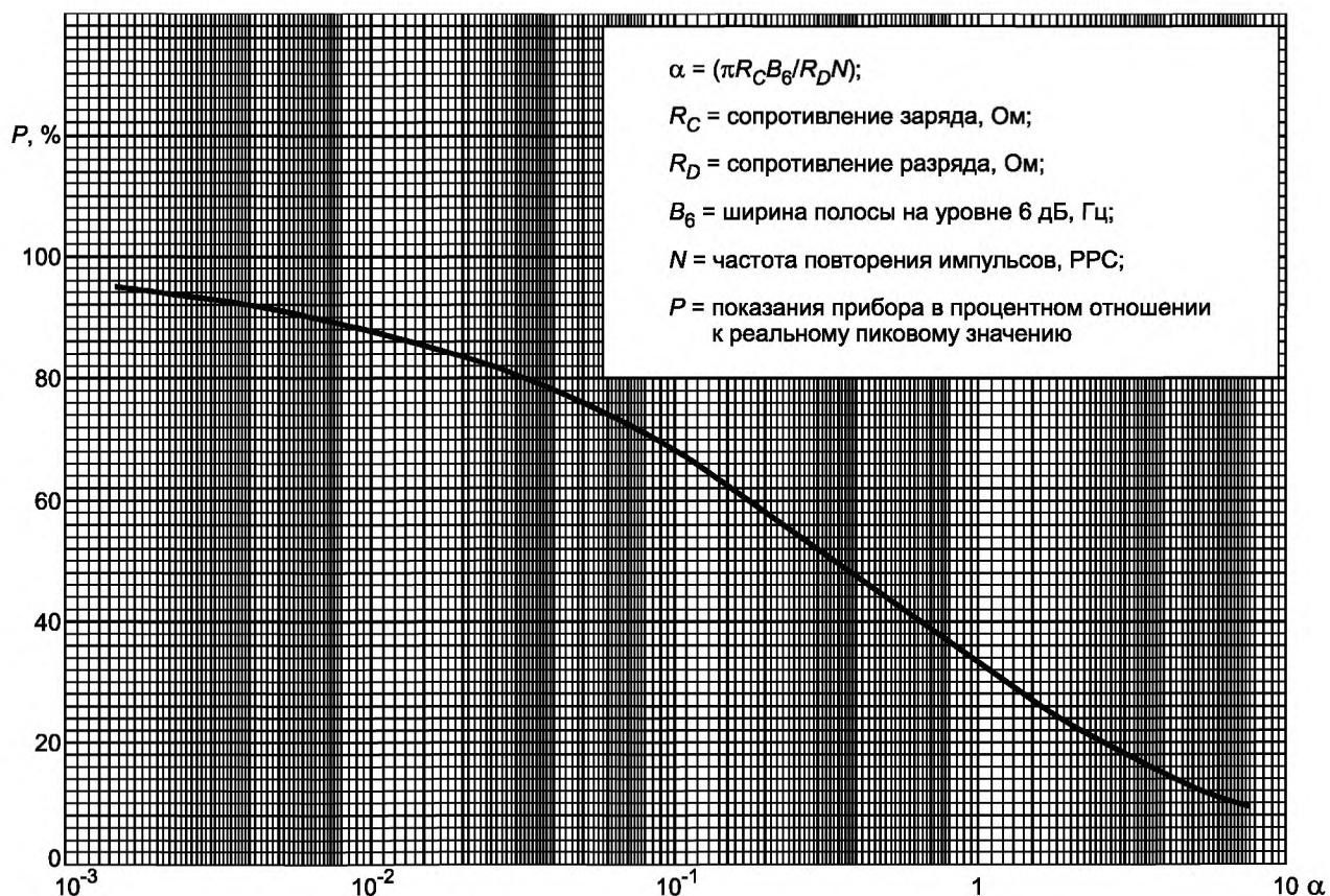
Рисунок Е.2 – Коэффициент выпрямления импульсов P (показания прибора в процентном отношении к реальному пиковому значению)
