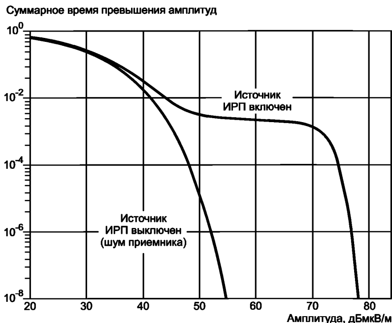
Рисунок G.3 — Пример функции распределения амплитуд ИРП
