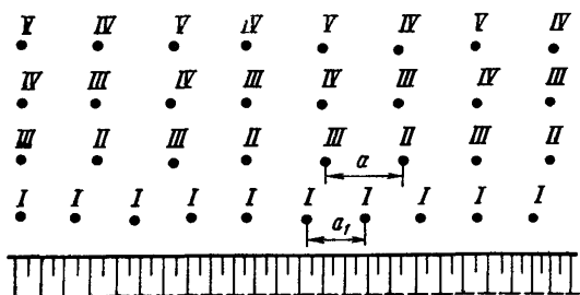
Рис. 66. Комбинированная схема КЗВ при завывенных СПШ первого ряда
