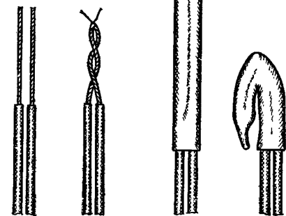
Рис. 55. Сращивание проводов и их изоляция при помощи шахтных зажимов
