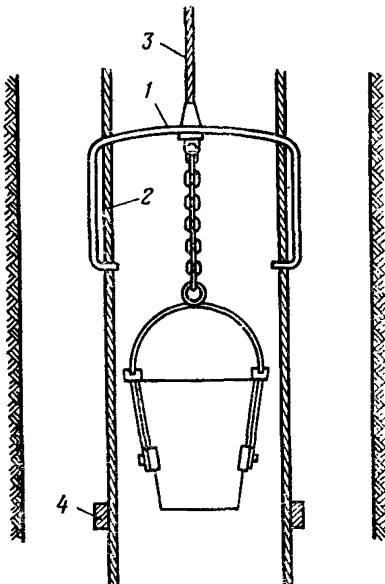
Рис. 4. Направляющее устройство для подъема бадь:
