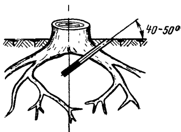
Рис. 38. Взрывание пней с разветвленной корневой системой
