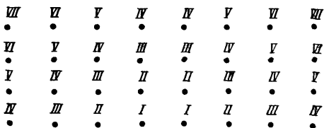
Рис. 63. Схема КЗВ «Трапециевидный вруб»
