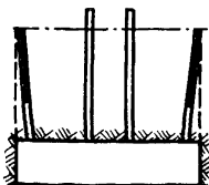
Рис. 24. Призматический вруб: 1 — заряжаемые шпурь; 2 — незаряжаемые шпурь
