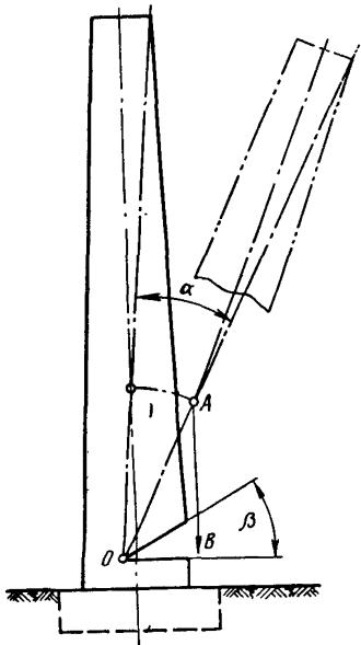
Рис. 36. Условие опрокидывания трубы в заданном направлении
