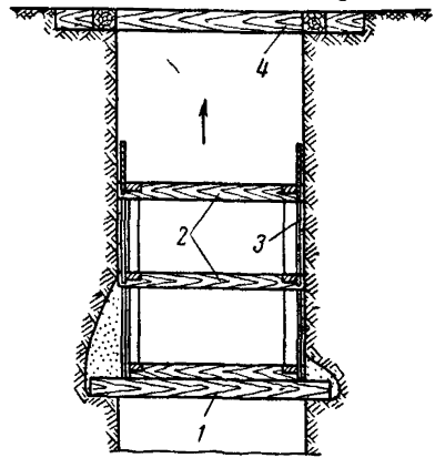
Рис. 17. Венцовая крепь на стойках:
