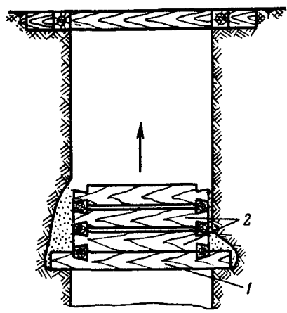
Рис. 15. Сплошная венцовая крепь, возводимая снизу вверх: 1 — основной венец; 2 — рядовые венцы
