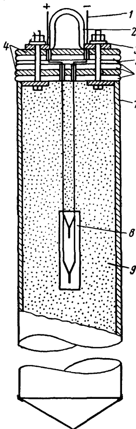
Рис. 44. Торпеда:
