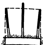
Рис. 25. Щелевой вруб: 1 — заряжаемые шпурь; 2 — незаряжаемые шпурь
