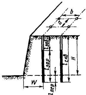
Рис. 8. Вертикальный скважинный заряд в уступе
