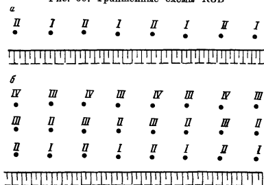
Рис. 61. Схема КЗВ через скважину: а — при однородном расположении скважин; б — при много- родном расположении скважин
