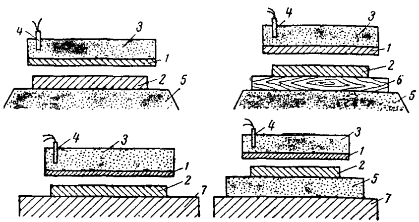
Рис. 47. Типы оснований при сварке металлов взрывом: 1 — перемещаемый элемент; 2 — неподвижный элемент; 3 — взрывчатое вещество; 4 — электродетонатор; 5 — песок; 6 — доска; 7 — металлическое основание
