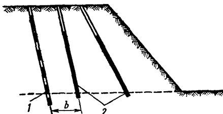
Рис. 16. Заряды: 1 — контурные; 2 — рыхления
