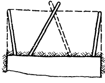
Рис. 23. Клиновой вруб «ножницы» (вертикальный)
