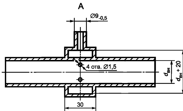
Деталь А
