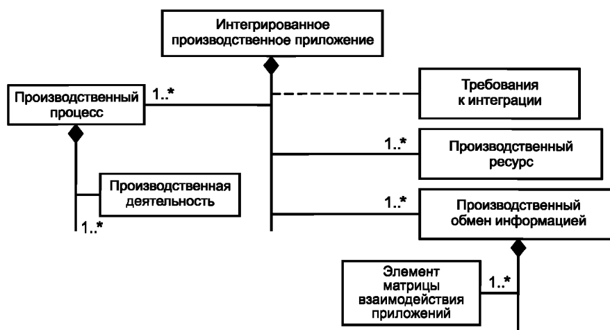
Рисунок 6 — Диаграмма соотношений интеграции приложений (AIRD)
