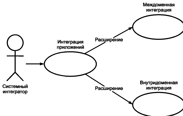
Рисунок 4 — Требования к интеграции приложений
