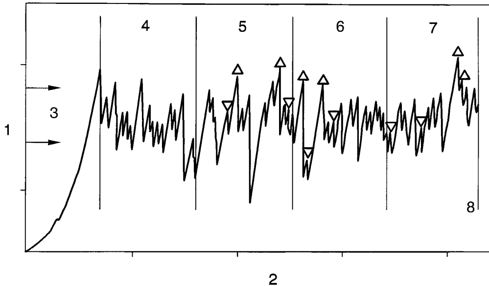
1 – усилие; 2 – направление раздирания (длина пути); 3 – аппроксимированный диапазон средних пиков; 4 – игнорировать; 5 – отрезок 1; 6 – отрезок 2; 7 – отрезок 3; 8 – конец разрыва
