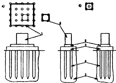
Рис. 7. Определение несущей способности армированного массива грунта (5) из НРС статическими испытаниями:
