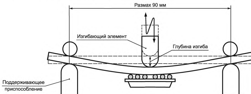
Рисунок 12 — Циклические испытания на прочность при изгибе
