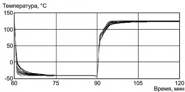
а) Распределение температуры (0 подложек)
