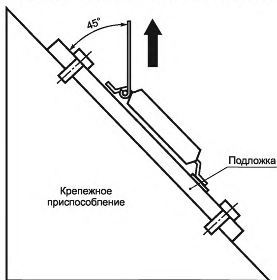
Рисунок 8 — Испытание прочности на отрыв
