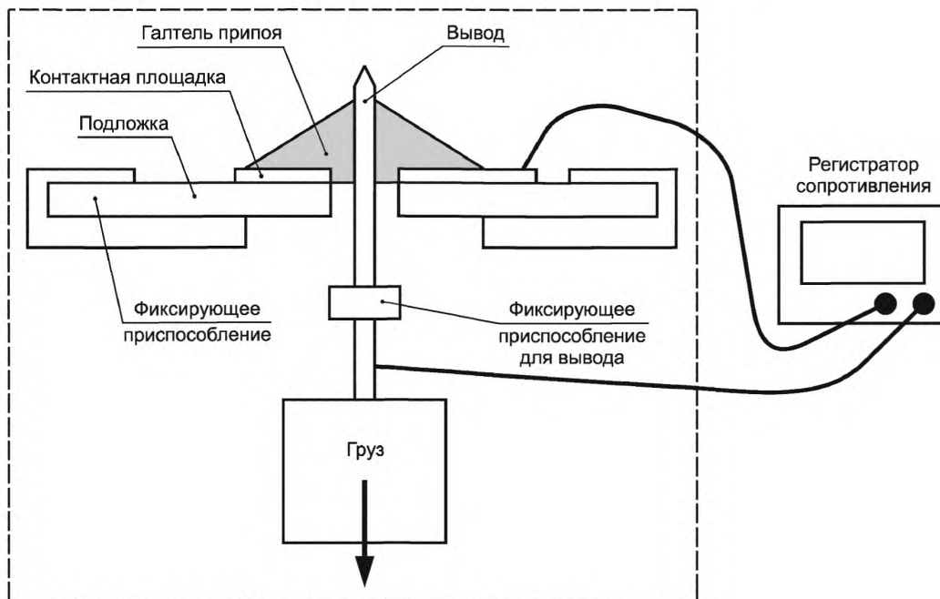
Рисунок 18 — Испытание на сопротивление ползучести
