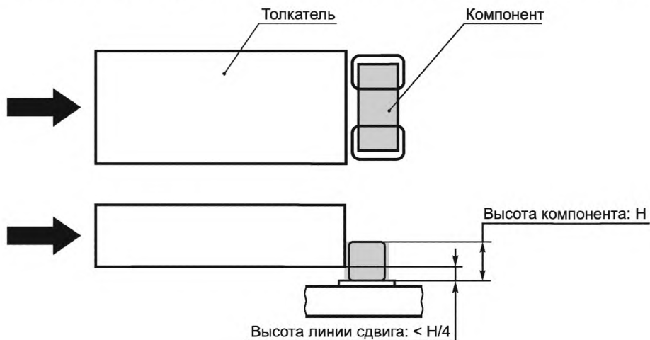
Рисунок 9 — Испытание прочности на сдвиг
