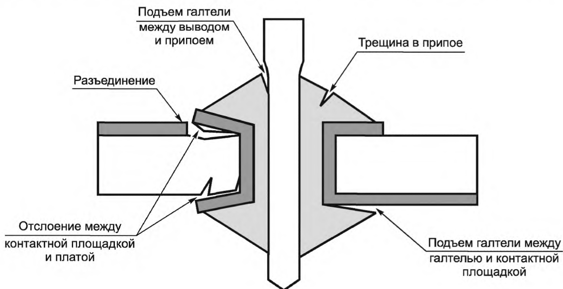
Рисунок Н.1 — Явление подъема галтели паяного соединения
