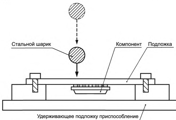
Рисунок 16 — Циклическое испытание на удар стальным шариком
