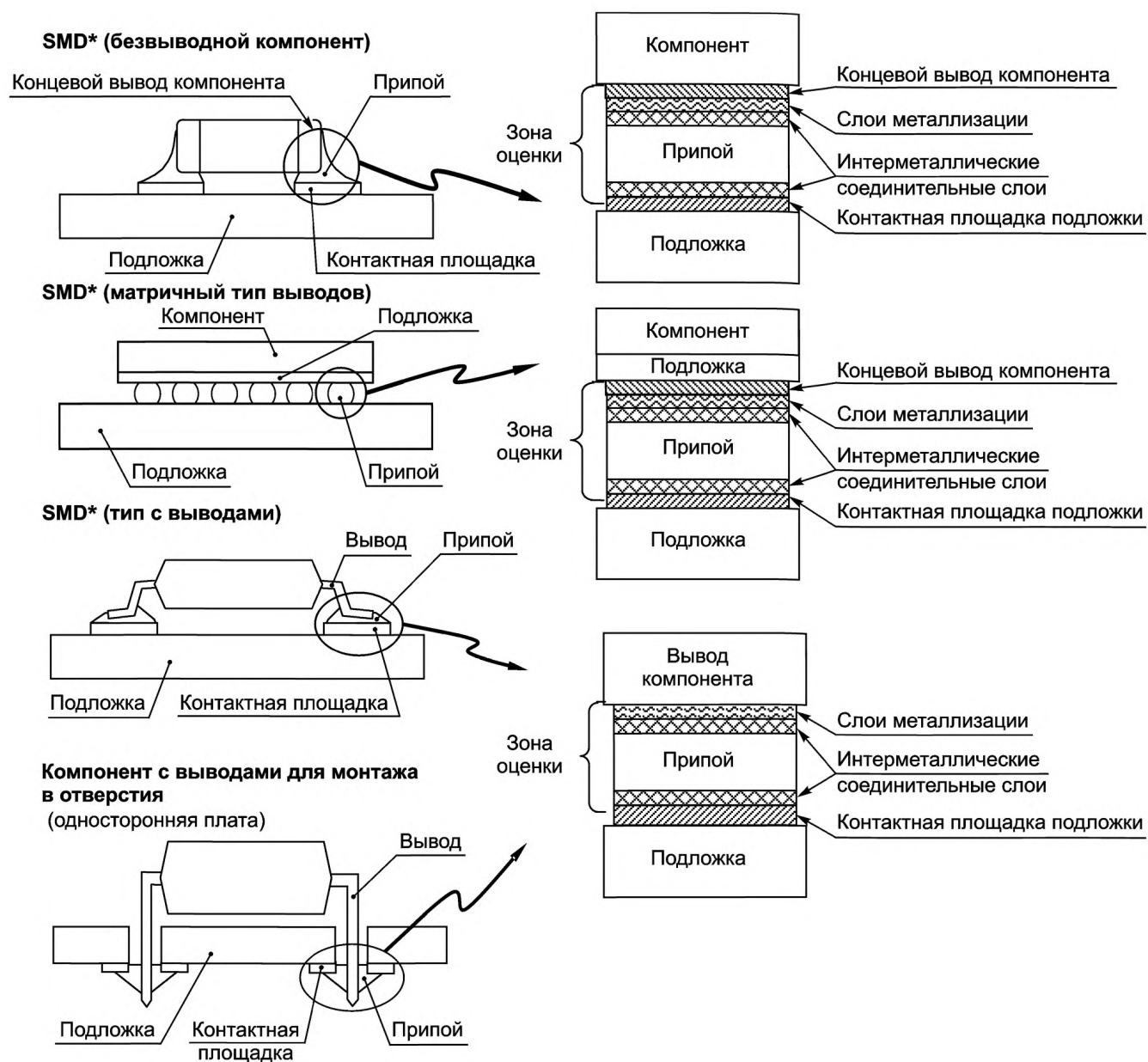
Рисунок 1 — Области соединений для испытаний на надежность
