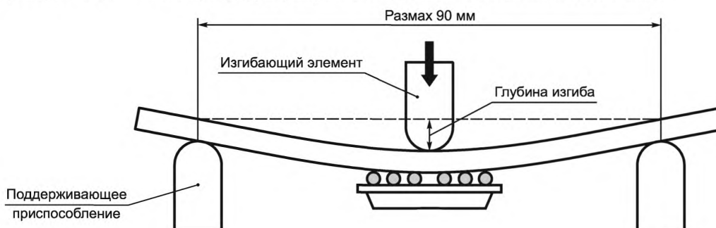
Рисунок 11 — Монотонное испытание на прочность при изгибе
