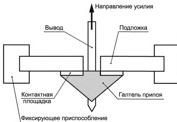
Рисунок 17 — Испытание прочности на отрыв
