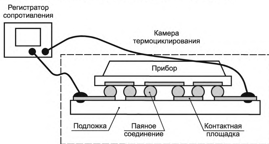
Рисунок В.1 — Пример схемы для проведения испытаний паяного соединения на наличие электрического соединения
