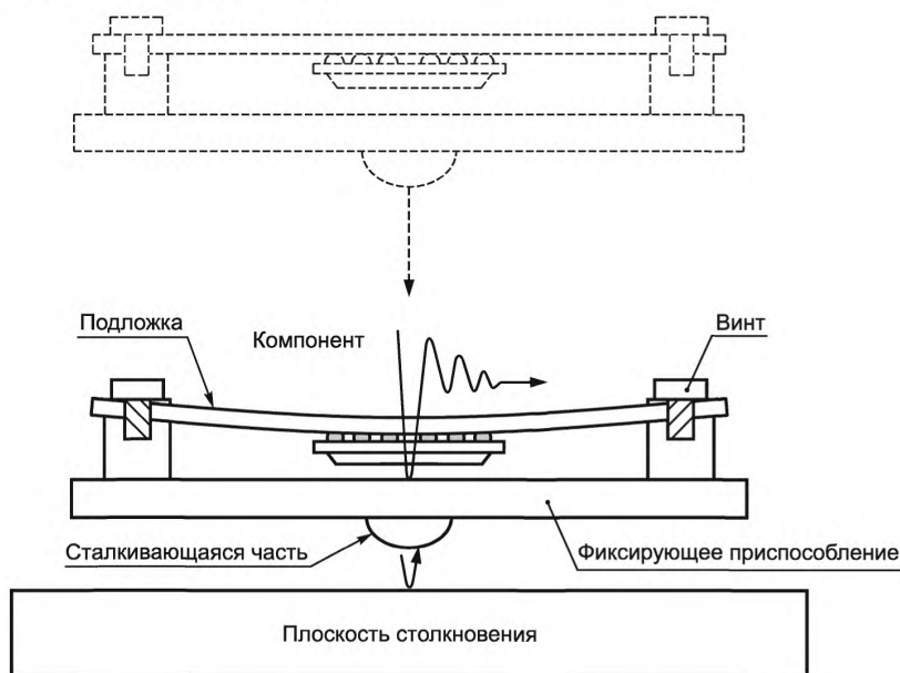
Рисунок 15 — Циклическое испытание на падение
