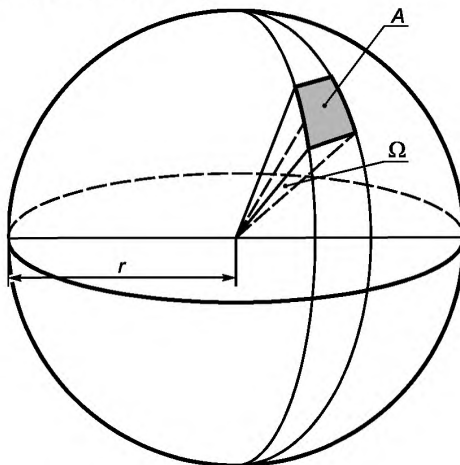
Рисунок 3 — Определение телесного угла
