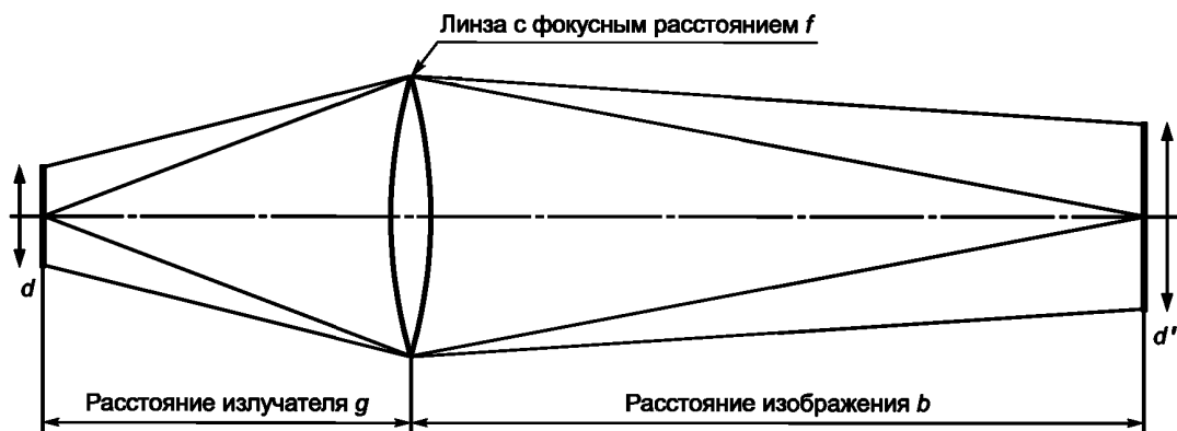
Рисунок 9 — Определение углового размера источника
