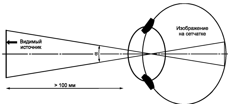
Рисунок 1 — Определение углового размера \alpha видимого источника
