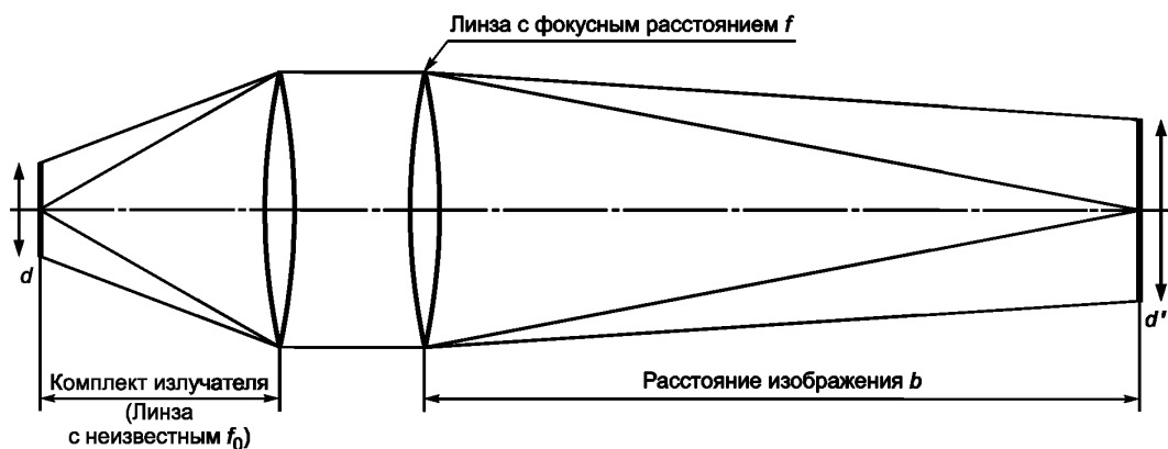
Рисунок 10 — Определение углового размера источника
