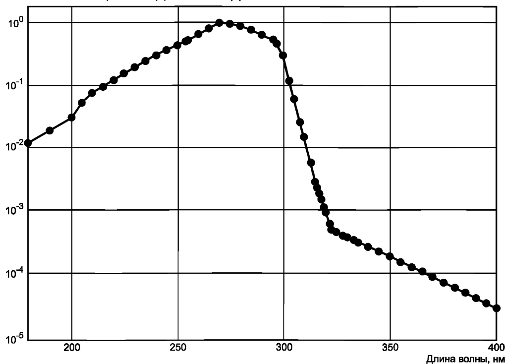
Относительная спектральная эффективность S(\lambda)
