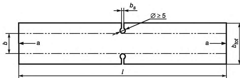
b — ширина испытываемого участка образца; b_{tot} — общая ширина образца; b_s — ширина паза
