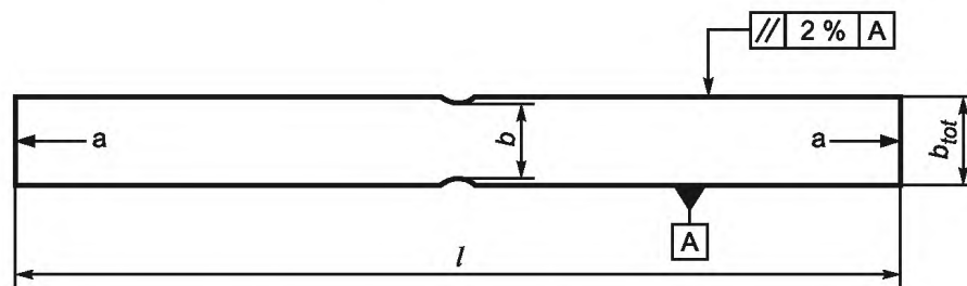
b — ширина испытываемого участка образца; b_{tot} — общая ширина образца
