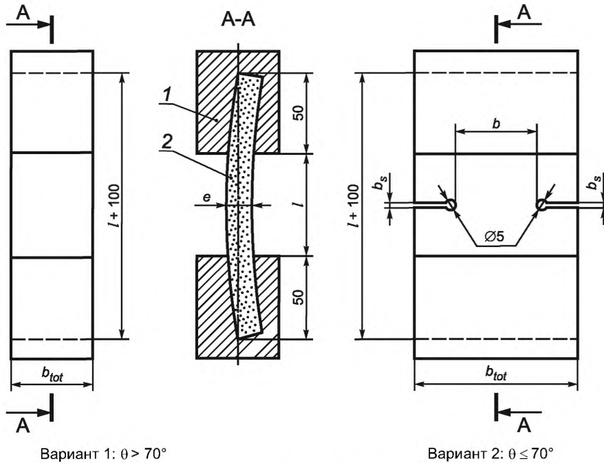
1 — конец образца, залитый смолой; 2 — образец; b_s — ширина паза; l — длина образца
