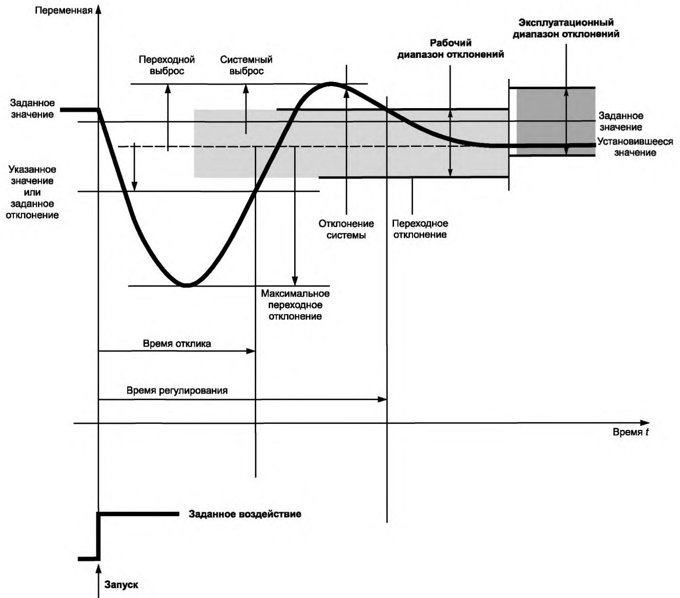
Рисунок D.4 — Переходный процесс при ступенчатом изменении нагрузки при постоянном опорном входном сигнале
