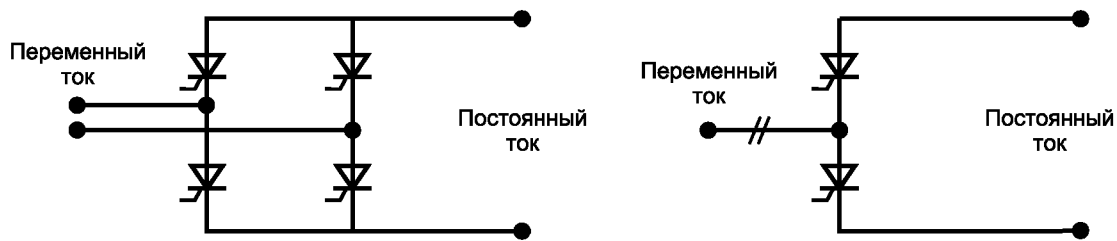
Пример однофазного моста Гретца
