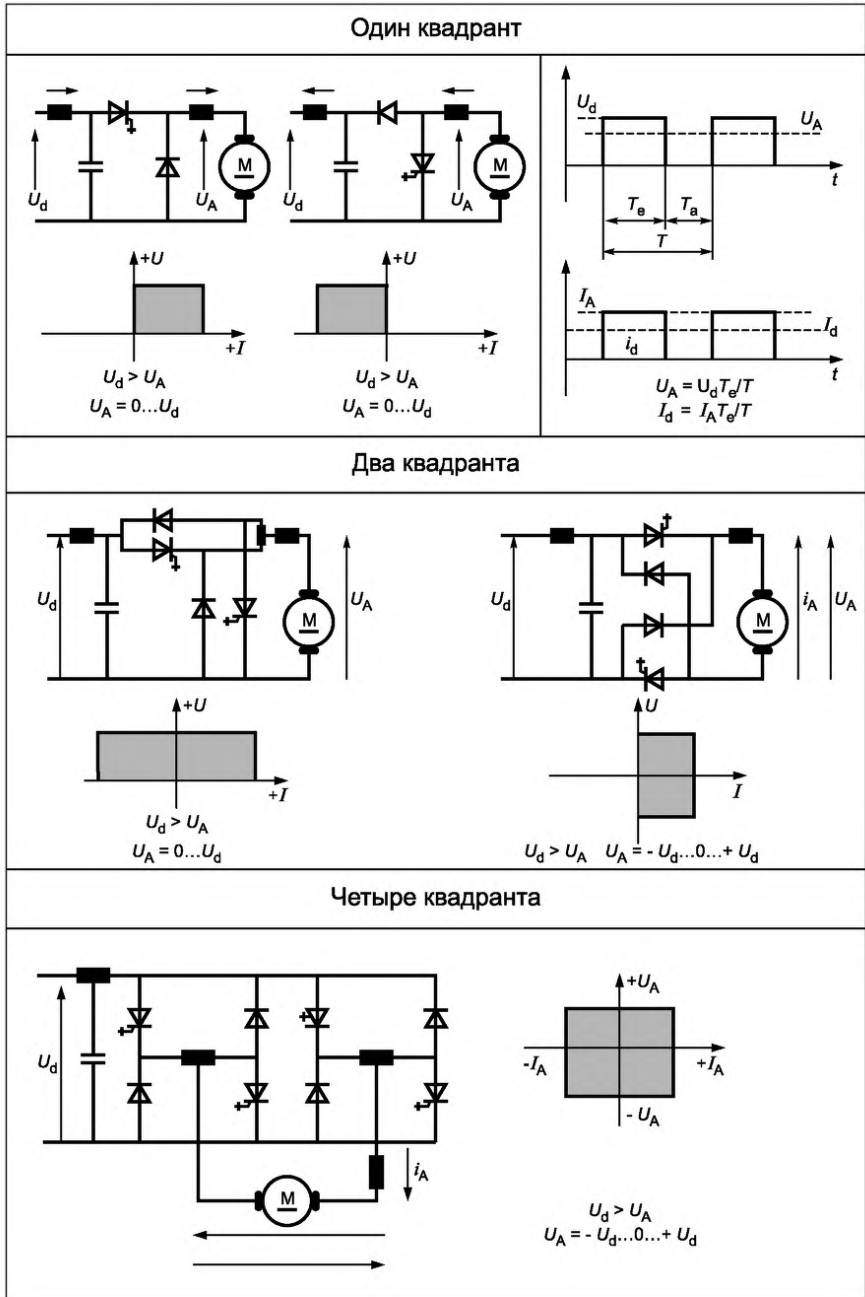
Рисунок F.2 — Преобразователи с внутренней коммутацией (прерыватели)
