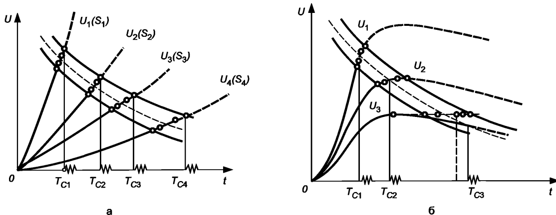
Рисунок 15 — Вольт-секундные характеристики изоляции
