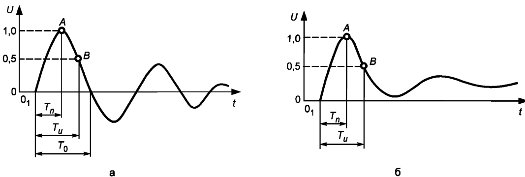
Рисунок 17 — Колебательный коммутационный импульс
