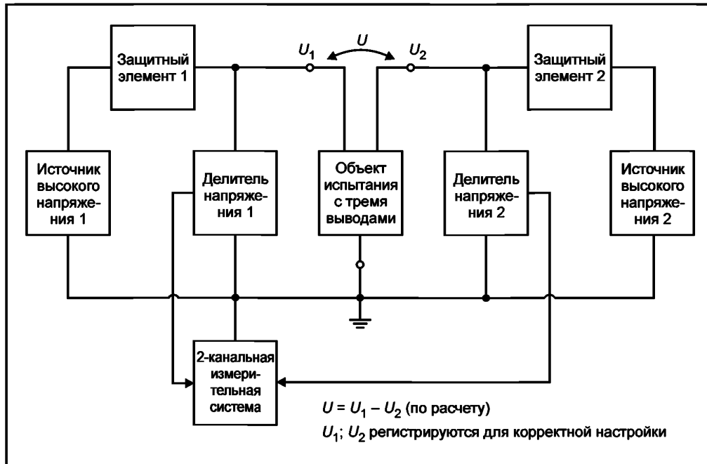
Рисунок 18 — Структурная схема испытаний комбинированным напряжением
