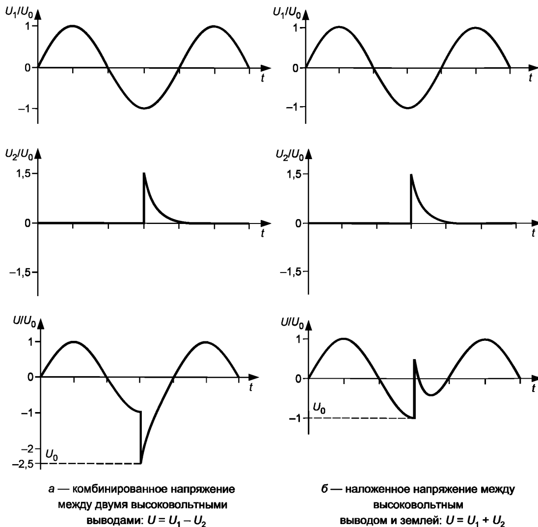
Рисунок 19 — Стилизованное представление комбинированного и наложенного напряжений
