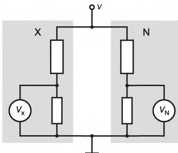
Рисунок Б.1 — Сличение испытываемой системы X с эталонной системой N
