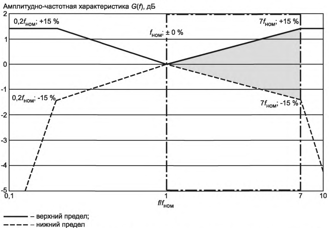
Рисунок 6 — Приемлемая нормализованная амплитудно-частотная характеристика измерительной системы (затемненная область), предназначенной для измерения одной из основных частот f_{\text{НОМ}} (испытанная в диапазоне 1-7 f_{\text{НОМ}} )
