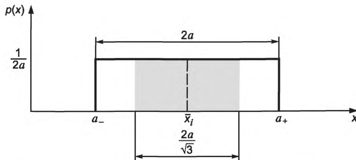
Рисунок А.2 — Плотность равномерного распределения вероятности p(x)
