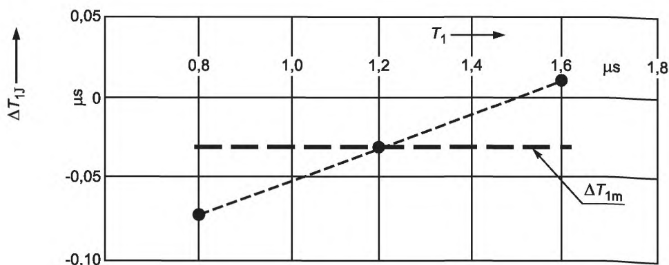
Рисунок Б.2 — Отклонение времени нарастания фронта (длительности переднего фронта) \Delta T_{1,j} измерительной системы X по отношению к эталонной измерительной системе N и их среднее значение \Delta T_{1m} в диапазоне T_1 = 0,8 \dots 1,6 мкс
