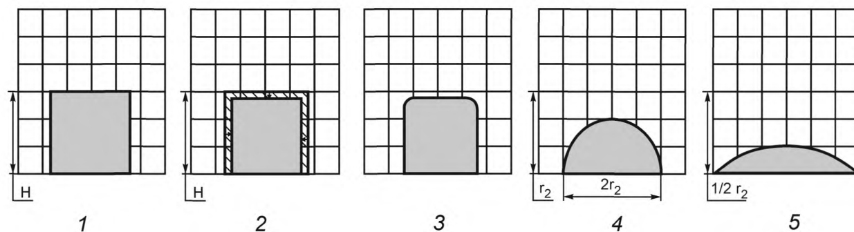
1 — исходный образец; 2 — усадка; 3 — деформация; 4 — полусфера; 5 — растекание
