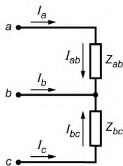
a, b, c — фазы основной вторичной обмотки ТН; I_a, I_b, I_c — фазные токи; I_{ab}, I_{bc} — междуфазные токи; Z_{ab}, Z_{bc} — междуфазные нагрузки
