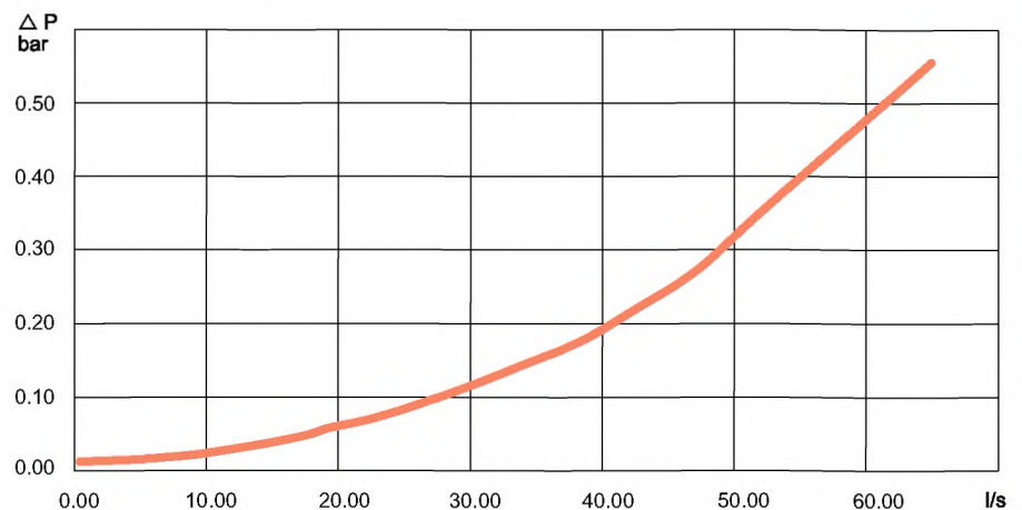
Расход воздуха при давлении на впуске 6,3 бар.
