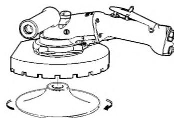
Комплект всасывания (для зачистки волоконным кругом)
