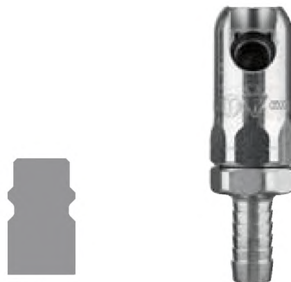
Профиль штуцера
