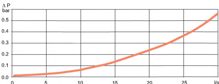
Расход воздуха при давлении на впуске 6,3 бар.
