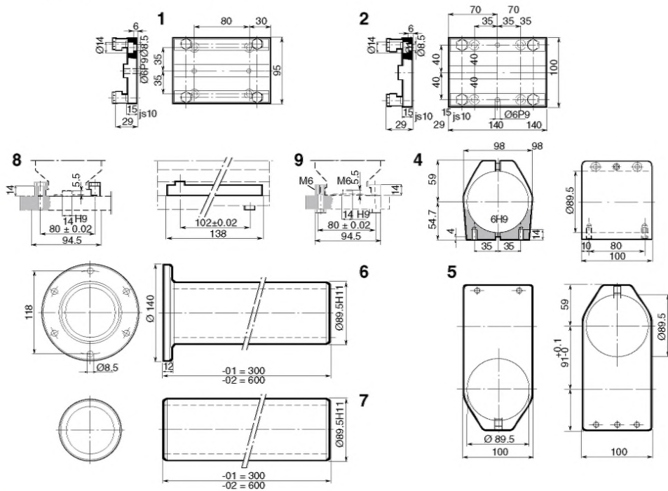
Чертеж с размерами – крепления для LBL45E
