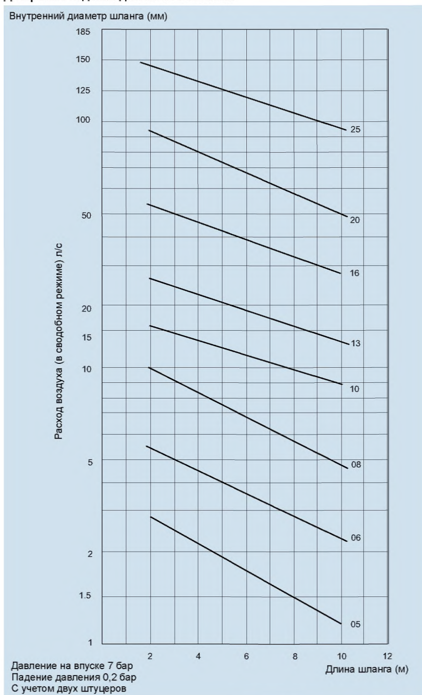
Диаграмма падения давления в шлангах
