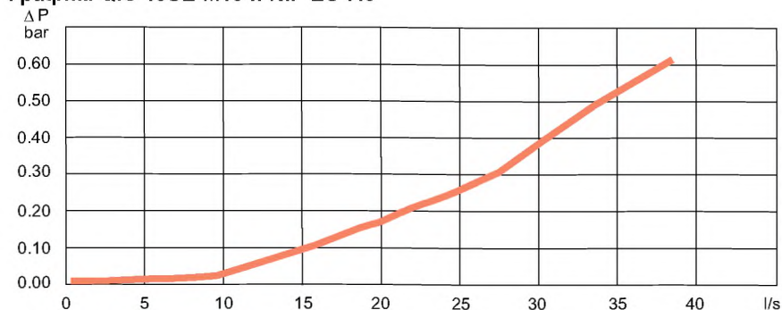
Расход воздуха при давлении на впуске 6,3 бар.
