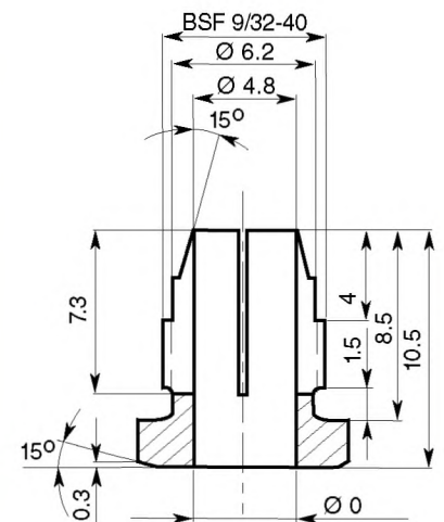
Цанги для 5,0 мм (Резьба BSF 9/32-40)
