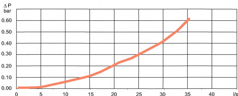
Расход воздуха при давлении на впуске 6,3 бар.
