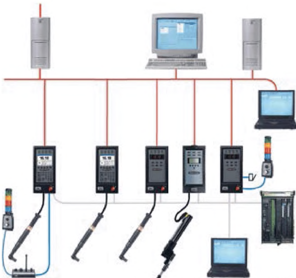
Дискретный ввод / вывод, шина ввода / вывода, Fieldbus, Compact, Graph, ПК, маршрутизатор доступа, база данных хоста.
