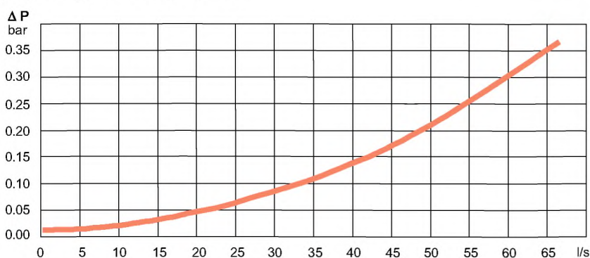
Расход воздуха при давлении на впуске 6,3 бар.
