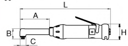
LBV11, -16, -36 90°
