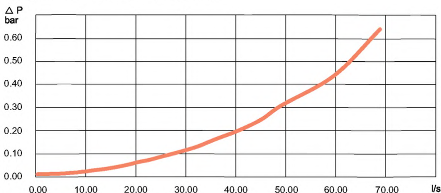
Расход воздуха при давлении на впуске 6,3 бар.
