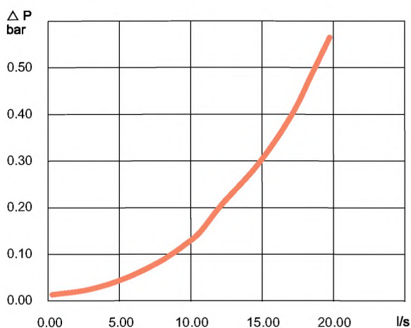
Расход воздуха при давлении на впуске 6,3 бар.
