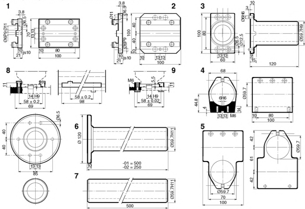
Чертеж с размерами – крепления для LBL25E и -35E
