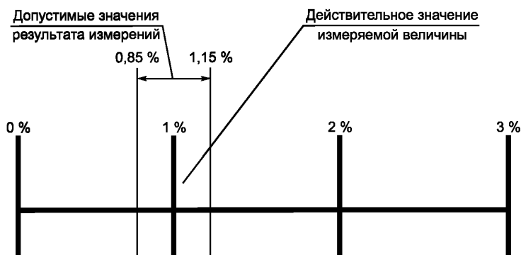
Рисунок 5 — Пример неопределенности измерений несимметрии напряжений
