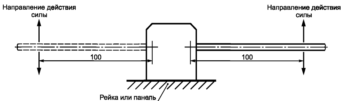
Рисунок 1 — Схема испытания по 8.3.2
