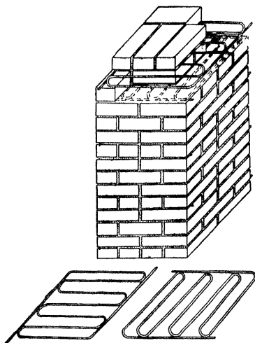
Рис. 6. Армирование кирпичных столбов сеткой «Зигзаг»
