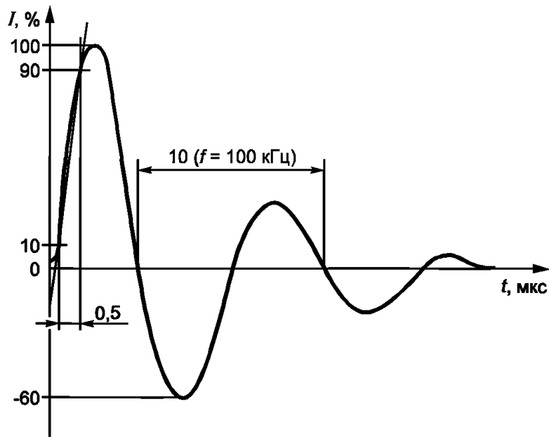
Рисунок 23 — Волнообразный импульс затухающего тока 0,5 мкс/100 кГц
