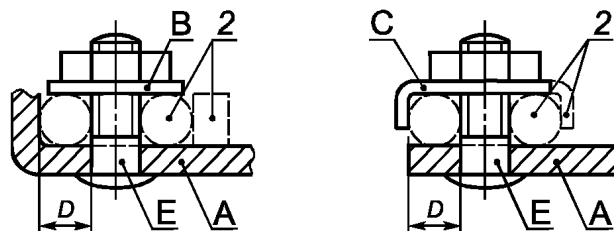
Рисунок IC.2b — Штыревые зажимы
