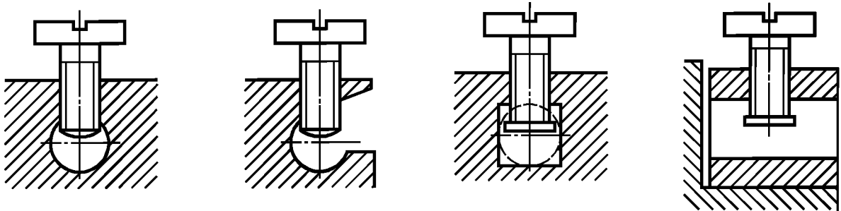
Рисунок IC.1b — Зажимы без прижимной пластины
