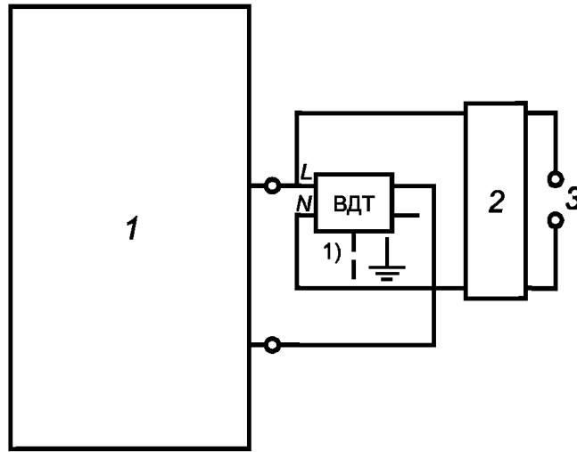
1 — генератор импульсного тока 8/20 мкс; 2 — фильтр; 3 — источник питания
