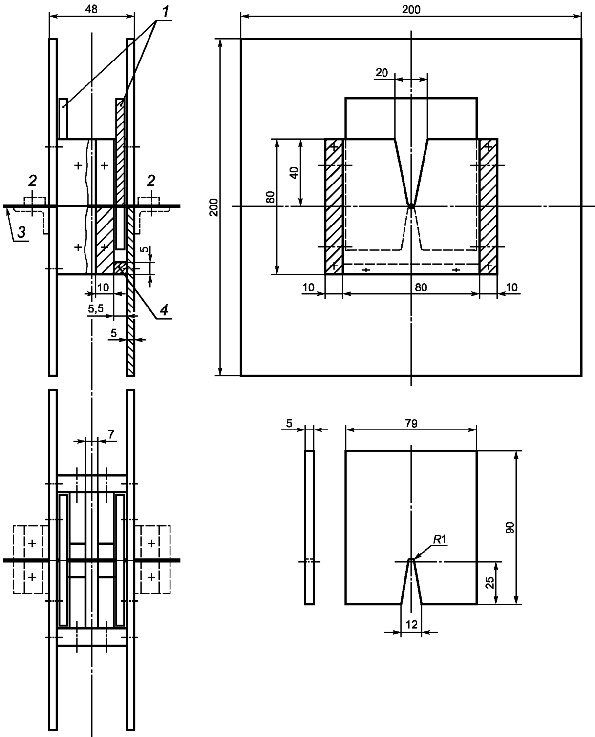
Рисунок 13 — Испытательное устройство для проверки минимальных значений I^2t и I_p , выдерживаемых ВДТ [9.11.2.1 а)]
