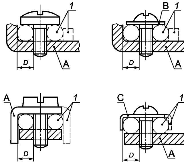
Рисунок IC.2a — Винтовые зажимы
