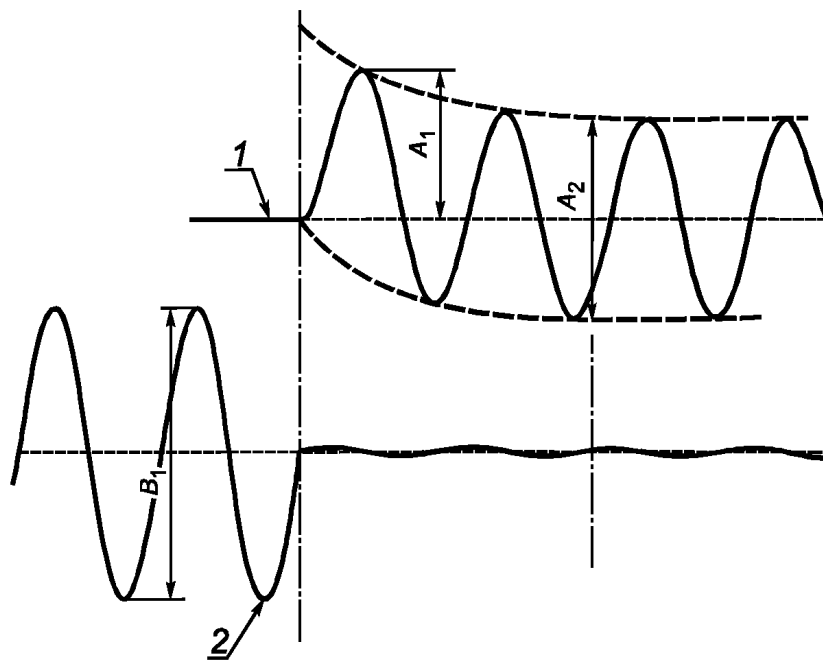
1 — ток; 2 — напряжение
