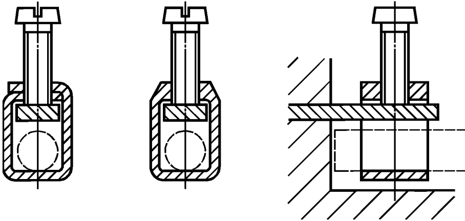
Рисунок IC.1a – Зажимы с хомутиком
