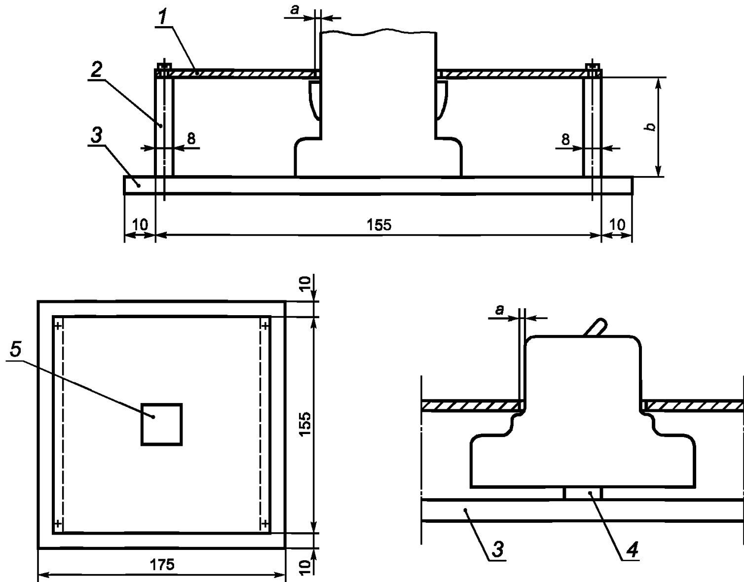
1 — съемная стальная пластина толщиной 1 мм; 2 — алюминиевые пластины; 3 — монтажная плита; 4 — планка для ВДТ; 5 — окно в стальной пластине для ВДТ
