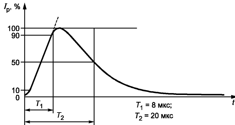
Рисунок 28 — Бросок импульсного тока 8/20 мкс
