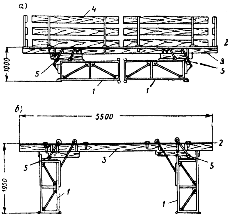
Рис. 37. Шарнирно-панельные подмости ППУ-4
