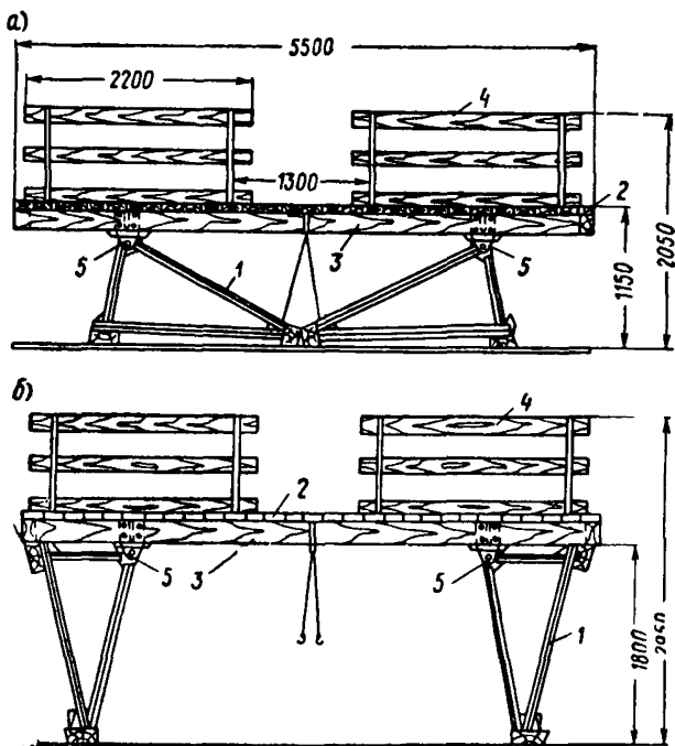
Рис. 35. Подмости треста № 94
