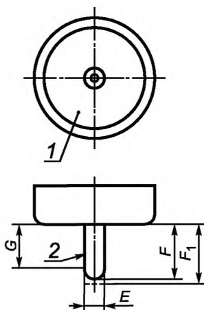
1 – изоляционный материал (вид произвольный); 2 – полированная поверхность для припайвания
