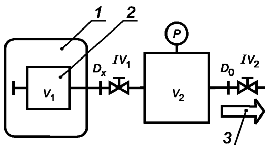
Рисунок Ж.1 — Схема испытания неповреждаемости
