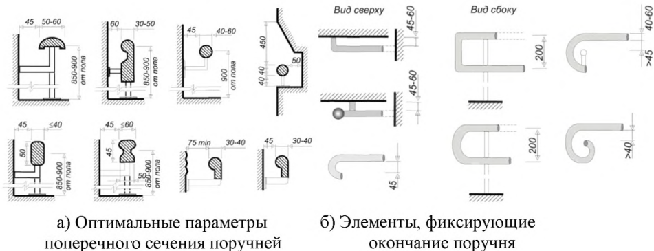
Рисунок 13 – Основные параметры конструкции поручней
