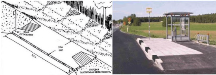
Рисунок 48 – Пример обустройства остановочного пункта пандусами
