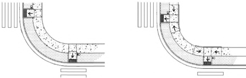
а) Типовое размещение пандуса в полосе озеленения
