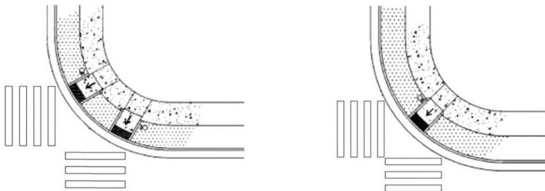
а) Применение пандусов на каждом пешеходном переходе
