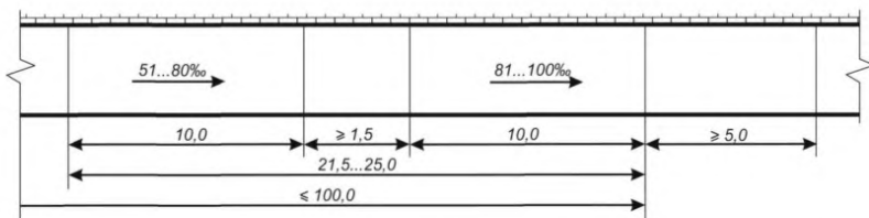
Рисунок 3 – Пример планировки тротуара (пешеходной дорожки) с продольным уклоном, соответствующим стесненным условиям движения инвалидов
