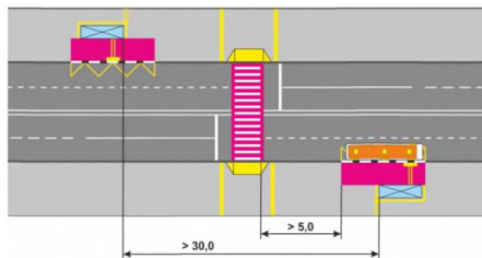
Рисунок 51 – Пример размещения остановочных пунктов, совмещенных с пешеходным переходом, доступным для инвалидов и других маломобильных групп населения
