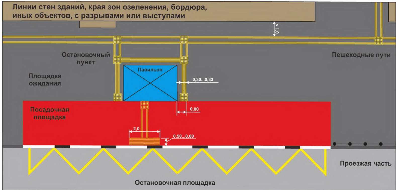
Рисунок Г.1 – Типовая схемы обустройства остановочного пункта и подходов к нему тактильными наземными указателями
