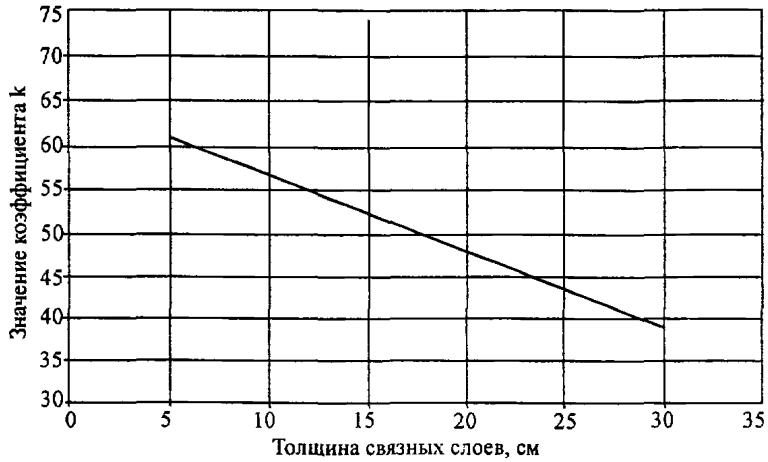
Рисунок 3 – График определения значений коэффициента k
