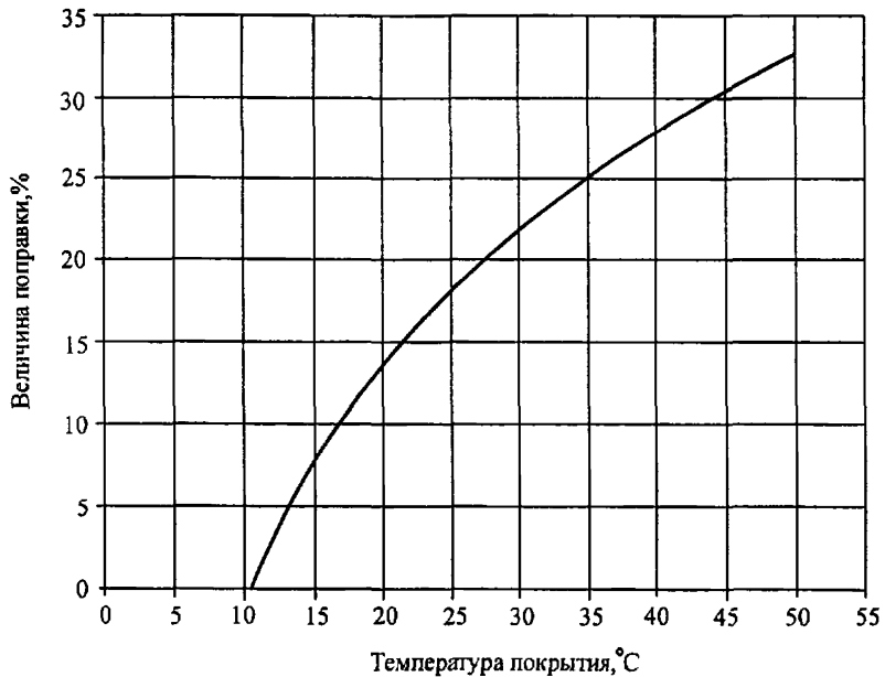
Рисунок 4 – График определения величины температурной поправки в полевых условиях в зависимости от толщины связных слоев
