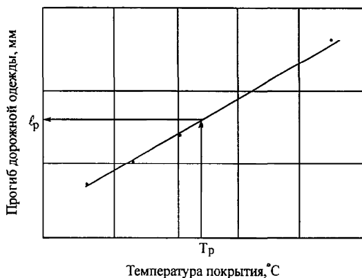
Рисунок 6 – Пример построения графика зависимости температуры покрытия от прогиба дорожной одежды по результатам испытания дорожной конструкции на контрольной точке
