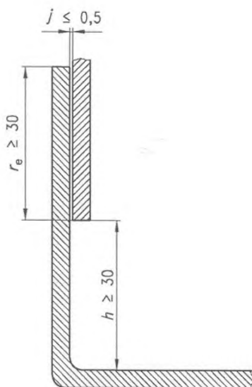
Рисунок В.5.3 – Зона разбрызгивания
