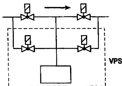
б – пример системы VPS с интегрированными клапанами
