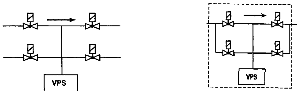
а – пример системы VPS с внешними клапанами
