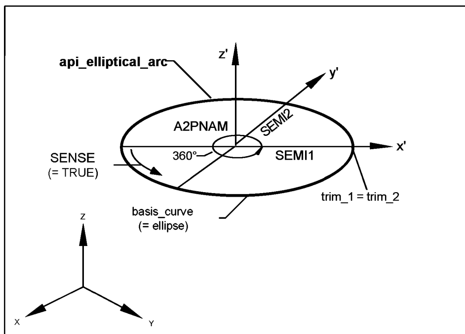
Api_elliptical_arc — результирующий эллипс; SEMI2 — малая полуось эллипса; A2PNAM — локальная координатная система; SENSE (= TRUE) — направление обхода — положительное (против часовой стрелки); SEMI1 — большая полуось эллипса; trim_1 = trim_2 — условие замкнутости кривой (начальная точка вычленения совпадает с конечной точкой вычленения); basis_curve (= ellipse ) — базовая кривая (эллипс)
