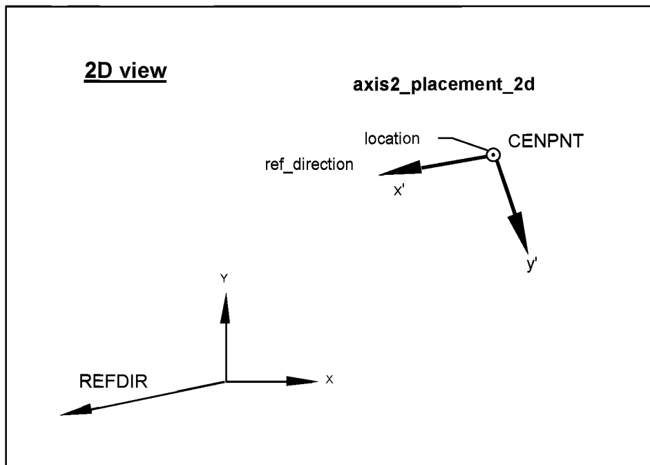
2D view — 2D-вид; axis2_placement_2d — сущность axis2_placement_2d ; location — размещение; CENPNT — начало координат; ref_direction — ссылочное направление; REFDIR — вектор базового направления
