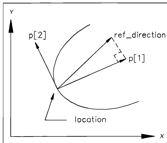
Ref_direction — ссылочное направление; location — вершина параболы
