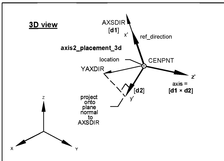
AXSDIR — вектор направления оси; 3D view — 3D-вид; ref_direction — ссылочное направление; axis2_placement_3d — сущность axis2_placement_3d ; location — размещение; CENPNT — начало координат; YAXDIR — имя аппроксимированного направления оси Y ; axis = [d1 x d2] — ось [d1 \times d2] ; project onto plane normal to AXSDIR — проекция на плоскость, перпендикулярную вектору направления оси
