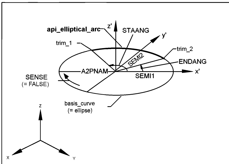
Api_elliptical_arc — результирующая дуга эллипса; STAANG — начальный угол дуги; trim_1 — первая точка вычленения; trim_2 — вторая точка вычленения; SEMI2 — малая полуось эллипса SEMI2; ENDANG — конечный угол дуги; A2PNAM — локальная координатная система; SEMI1 — большая полуось эллипса SEMI1; SENSE (= FALSE) — направление обхода дуги — отрицательное (по часовой стрелке); basis_curve (= ellipse) — базовая кривая (эллипс)
