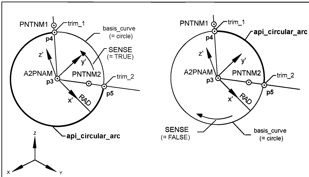
PNTNM1 — первая заданная точка; trim_1 — первая точка вычленения; basis_curve (= circle) — базовая кривая (окружность); api_circular_arc — построенная дуга окружности; SENSE (= TRUE) — обход кривой в положительном направлении; A2PNAM — начало локальной координатной системы; PNTNM2 — вторая заданная точка; trim_2 — вторая точка вычленения; RAD — радиус; SENSE (= FALSE) — обход кривой в отрицательном направлении
