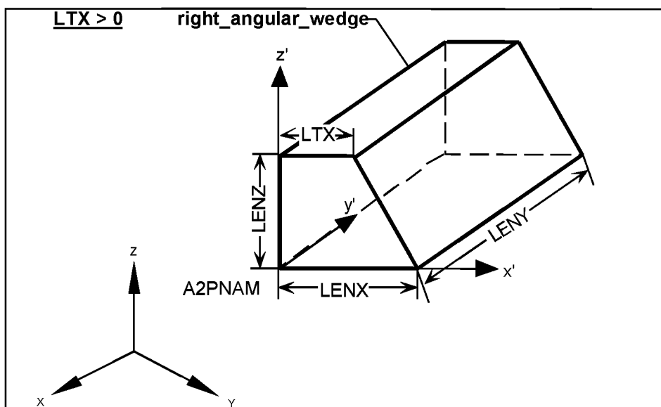
Рисунок А.43 — Функция Wdg_Gen
