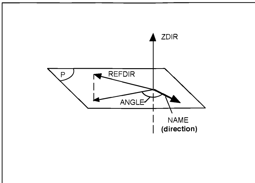
Рисунок А.2 — Функция Dir_2_Dir_Angle
