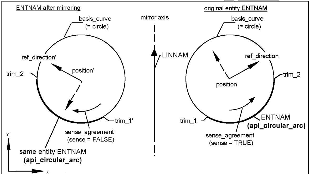
ENTNAM after mirroring — зеркально отраженная сущность; original entity ENTNAM — прообраз исходной сущности; basis_curve (= circle) — базовая кривая (окружность); mirror axis — ось зеркального отражения; ref_direction' — ссылочное направление; LINNAM — прямая с именем LINNAM; ref_direction — ссылочное направление; trim_2' — вторая точка вычленения; position' — зеркально отраженное начало координат; trim_2 — вторая точка вычленения; position — зеркально отраженное начало координат; ENTNAM — дуга окружности ENTNAM; trim_1' — первая точка вычленения; trim_1 — первая точка вычленения; api_circular_arc — сущность дуги окружности; sense_agreement (sense = FALSE) — отрицательное направление обхода кривой (значение атрибута sense равно «false»); sense_agreement (sense = TRUE) — положительное направление обхода кривой (значение атрибута sense равно «true»); same entity ENTNAM — зеркально отраженная дуга окружности ENTNAM
