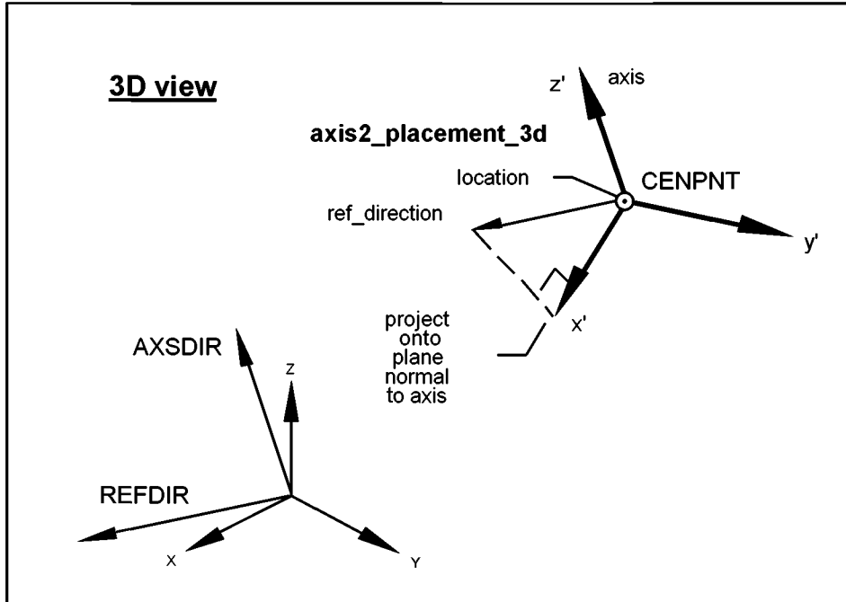
Axis — ось; 3D view — 3D-вид; axis2_placement_3d — сущность axis2_placement_3d ; location — размещение; CENPNT — начало координат; ref_direction — ссылочное направление; project onto plane normal to axis — проекция на плоскость, перпендикулярную оси; AXSDIR — вектор направления оси; REFDIR — вектор базового направления
