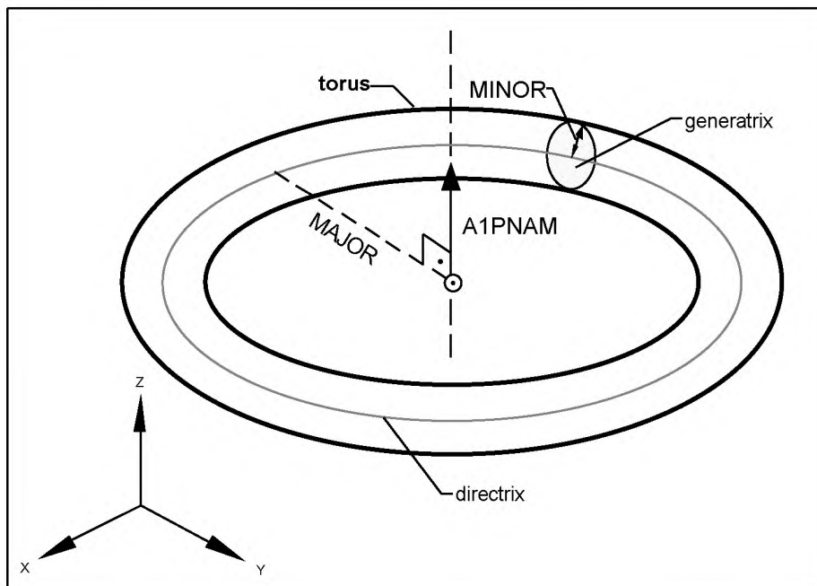
Torus — тор; MINOR — радиус образующей окружности; generatrix — образующая линия; A1PNAM — локальная координатная система; MAJOR — радиус направляющей окружности; directrix — направляющая линия
