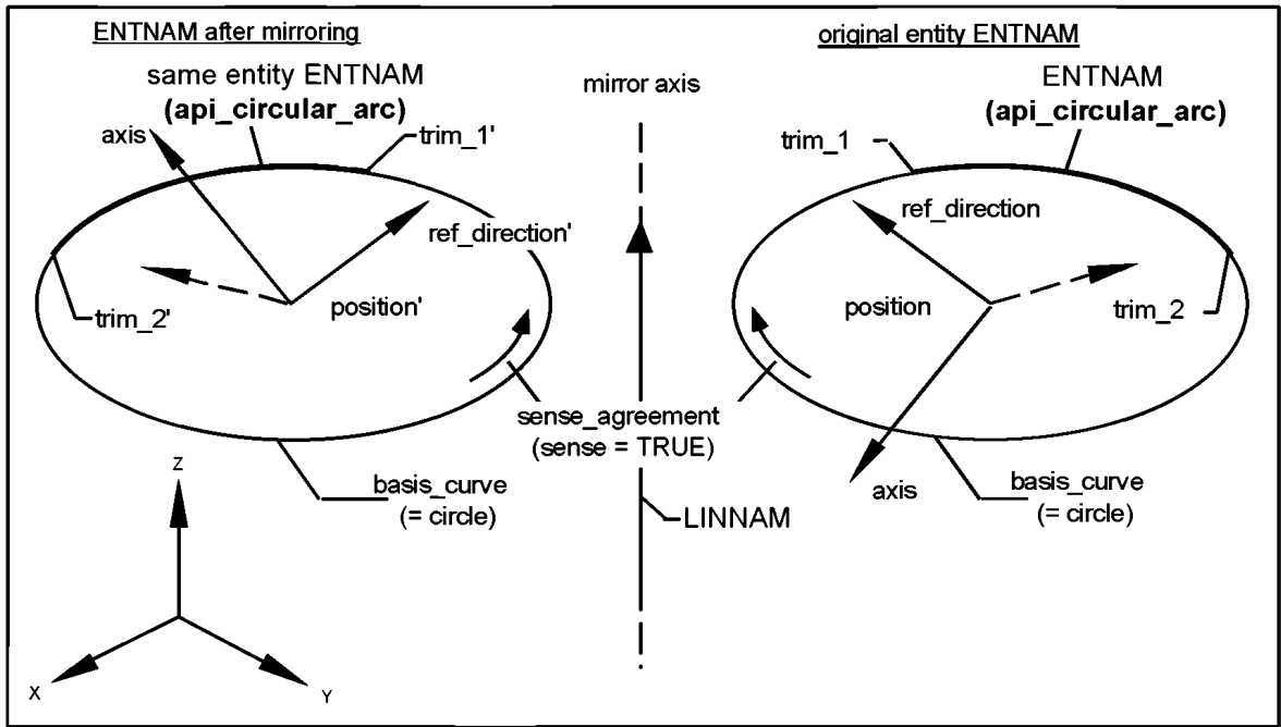
ENTNAM after mirroring — зеркально отраженная сущность; original entity ENTNAM — прообраз исходной сущности; same entity ENTNAM — зеркально отраженная дуга окружности ENTNAM; mirror axis — ось зеркального отражения; ENTNAM — исходная сущность; api_circular_arc — примитив дуги окружности; trim_1' — первая точка вычленения; trim_1 — первая точка вычленения; ref_direction' — ссылочное направление; ref_direction — ссылочное направление; position' — зеркально отраженное начало координат; position — зеркально отраженное начало координат; trim_2' — вторая точка вычленения; trim_2 — вторая точка вычленения; sense_agreement (sense = TRUE) — положительное направление обхода кривой (значение атрибута sense равно «true»); basis_curve (= circle) — базовая кривая (окружность); axis — ось; LINNAM — прямая с именем LINNAM
