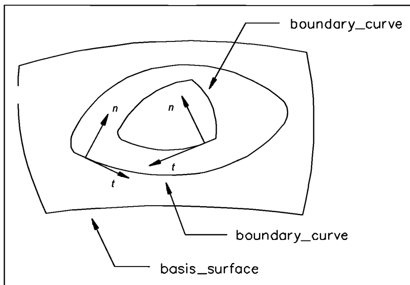
Boundary_curve — ограниченная кривая; basis_surface — базовая поверхность
