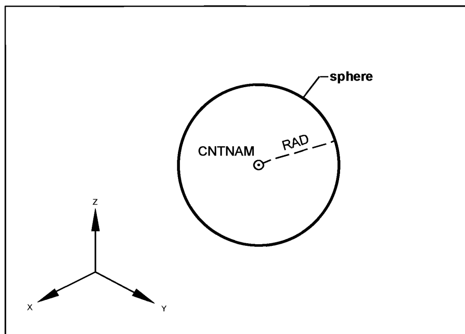
Рисунок А.38 — Функция Sph_Gen
