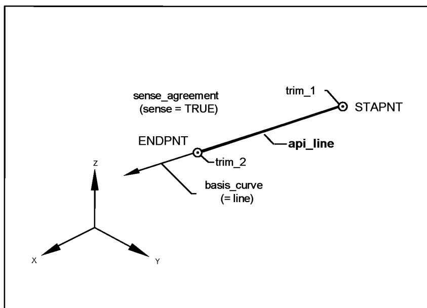
Trim_1 — точка вычленения 1; sense_agreement (sense = TRUE) — положительное направление отрезка (совпадает с направлением оси); STAPNT — начальная точка отрезка; ENDPNT — конечная точка отрезка; api_line — сущность линии; trim_2 — точка вычленения 2; basis_curve (= line) — базовая кривая (прямая линия)
