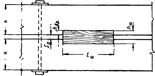
Рис. 13. Схема соединения на деревянных колодках
