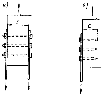
Рис. 16. Нагельные соединения со стальными накладками а — двусторонние; б — односторонние
