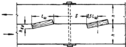
Рис. 12. Схема соединения на деревянных наклонных прямоугольных шпонках
