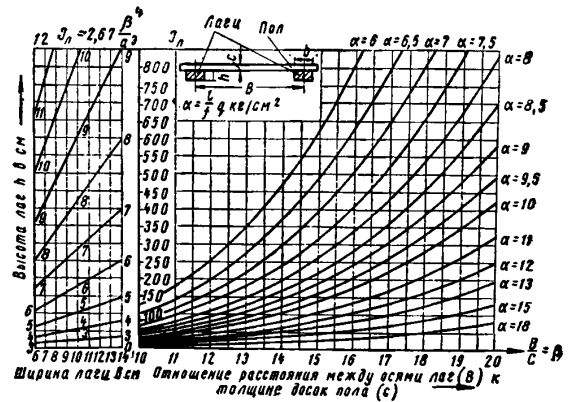
Рис. 23. График для расчета деревянных перекрытий на зыбкость
