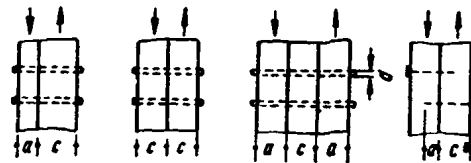
Рис. 15. Несимметричные соединения на нагелях
