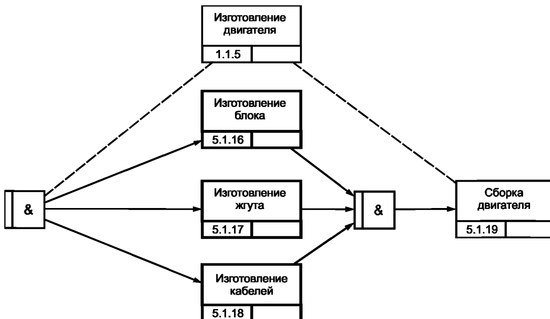
Рисунок В.2 — Процесс изготовления двигателя изделия GT-350 [4]
