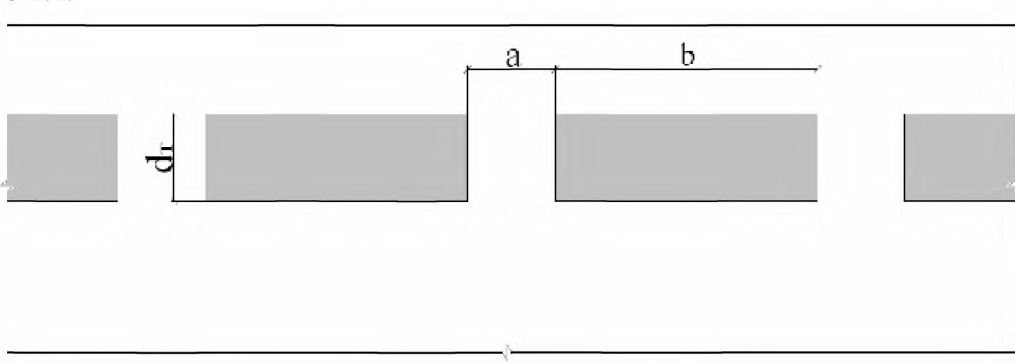
Рис. Е.1 Схема перфорации плиты перекрытия.
