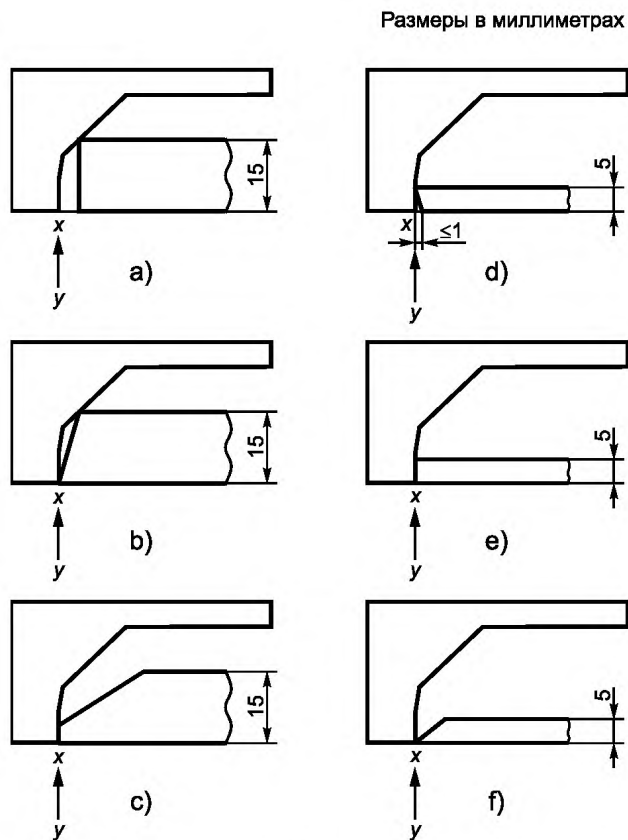
Случаи a) и b) — не соответствуют; случаи c), d), e) и f) — соответствуют (соответствие должно быть проверено требованиями 20.8, используя калибр, представленный на рисунке 23)
