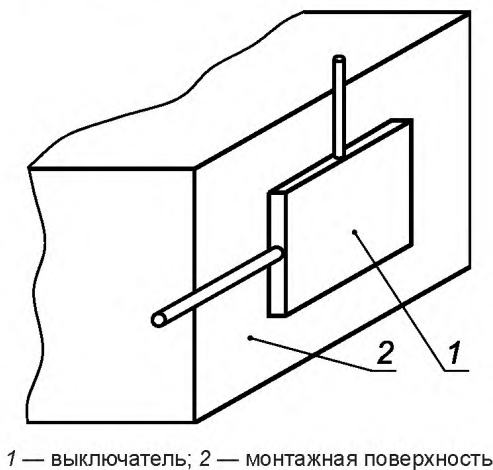
Рисунок 24 — Схема, показывающая направление приложения калибра согласно рисунку 23
