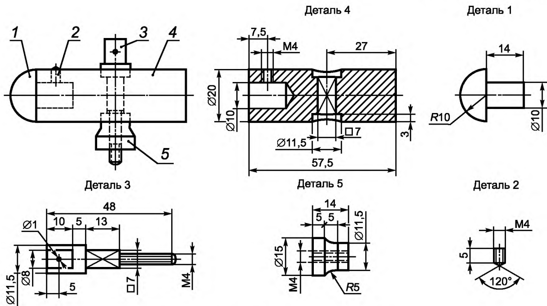
Рисунок 16 — Устройство маятника для испытания на удар
