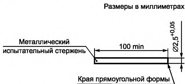
Рисунок 23 — Калибр для проверки пазов, отверстий и обратных конусов
