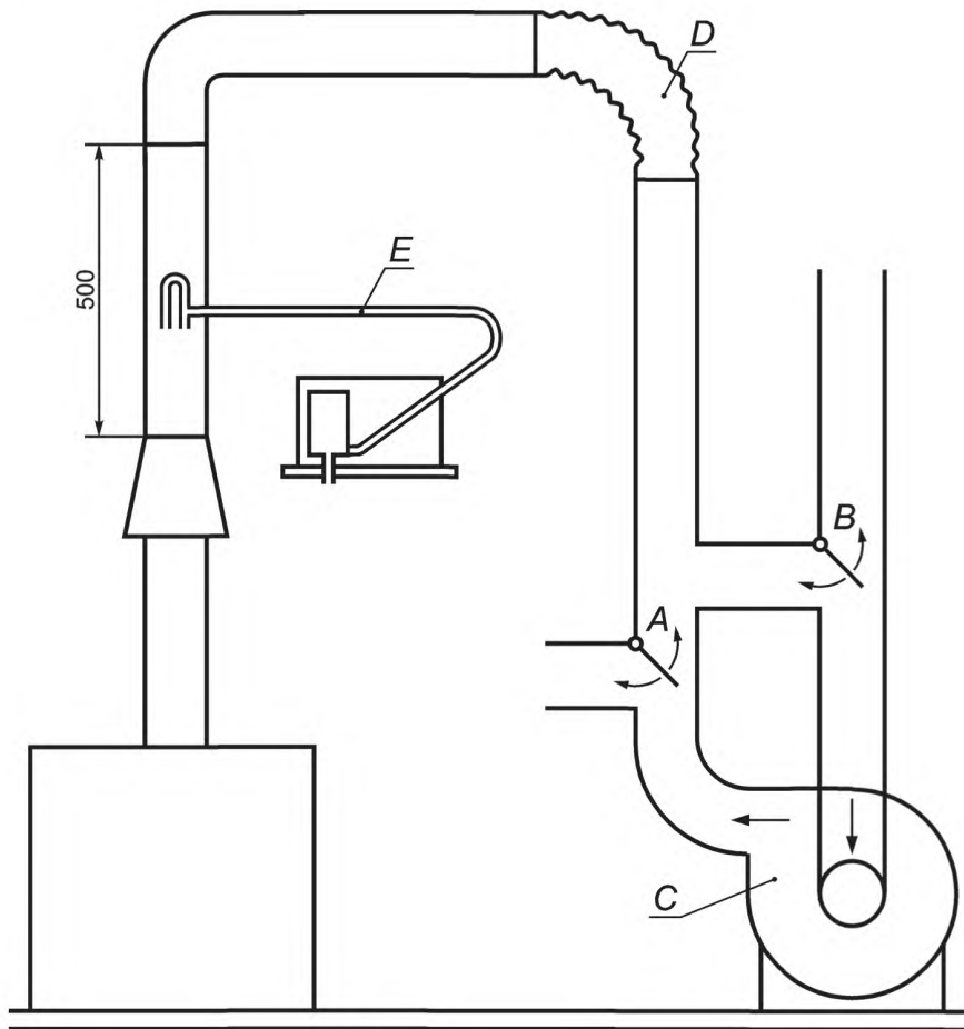
A и B — пропускные клапаны для получения восходящей и обратной тяги; C — вентилятор; D — гибкий участок; E — измерение скорости с помощью трубки Пито
