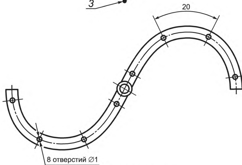
1 — медная трубка \varnothing 6 мм; 2 — медная трубка \varnothing 4,3 мм; 3 — термопара Рисунок 10 — Пробоотборник для отбора проб продуктов сгорания для испытательных дымоходов диаметром D < 100 мм
