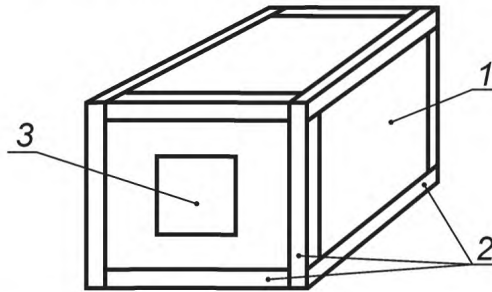
1 — защитная оболочка; 2 — рама из уголка 40 × 40 мм; 3 — крышка испытуемого образца
