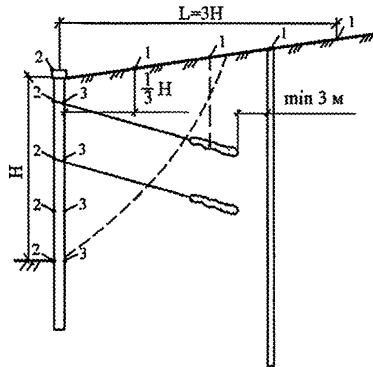
1; 2 – геодезические марки; 3 – датчики давления грунта и порового давления; H – высота удерживаемого массива грунта, м; L – максимальное расстояние установки геодезических марок, м Рисунок 25 – Рекомендуемая схема расстановки точек наблюдения
