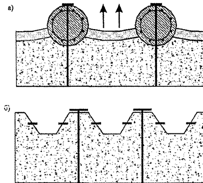
Рисунок 16 – Сопряжение через центр рабочей сваи
