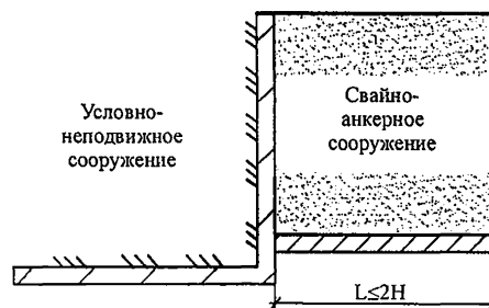
Рисунок 7 – Форма внутреннего угла подпорной стены
