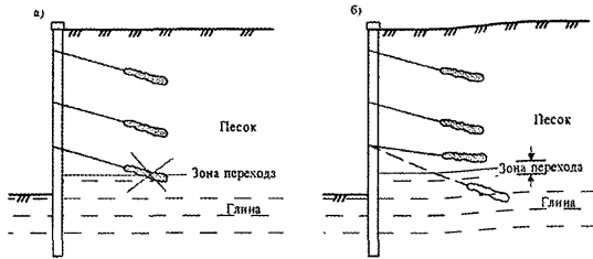
Рисунок 22 – Расположение анкеров на границе инженерно-геологических элементов
