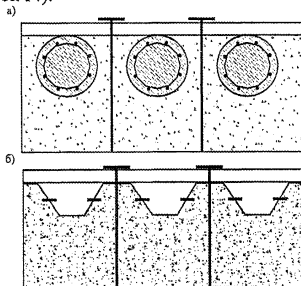
а – буровые сваи; б – шпунт
