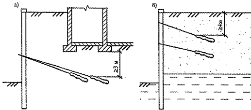
Рисунок 18 – Минимальное расстояние (а, б) до корня анкера
