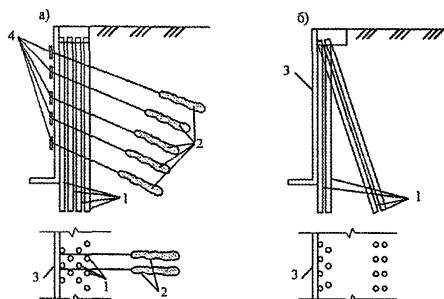
Рисунок 23 – Устройство многорядных свайных стен из буроинъекционных вертикальных свай (а) и вертикальных и наклонных свай (б)
