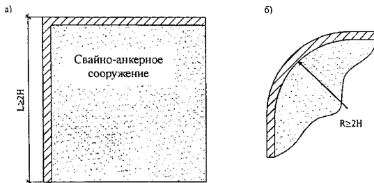
H – высота удерживаемого массива грунта, м; L – протяженность сооружения, м; R – радиус поворота сооружения, м Рисунок 5 – Формы сооружения в плане (а, б), образующие внешний угол
