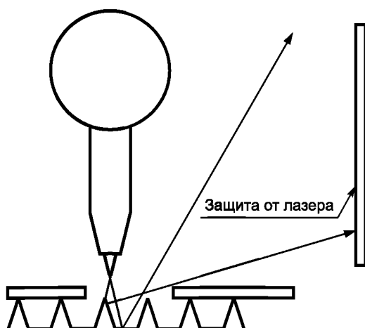
Рисунок В.3с — Отсутствие заготовки
