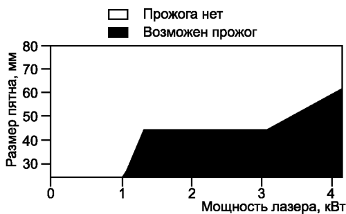
Рисунок F.20 — Стойкость к разрушению листа алюминия толщиной 2 мм от 100 с экспозиции расфокусированного пучка во время экспериментов с использованием непрерывного лазера на иттрий-алюминиевой гранате с неодимом
