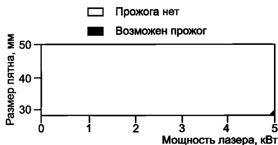
Рисунок F.11 — Стойкость к разрушению листа поликарбоната толщиной 6 мм от 10 с экспозиции расфокусированного пучка во время экспериментов с использованием непрерывного лазера на углекислом газе
