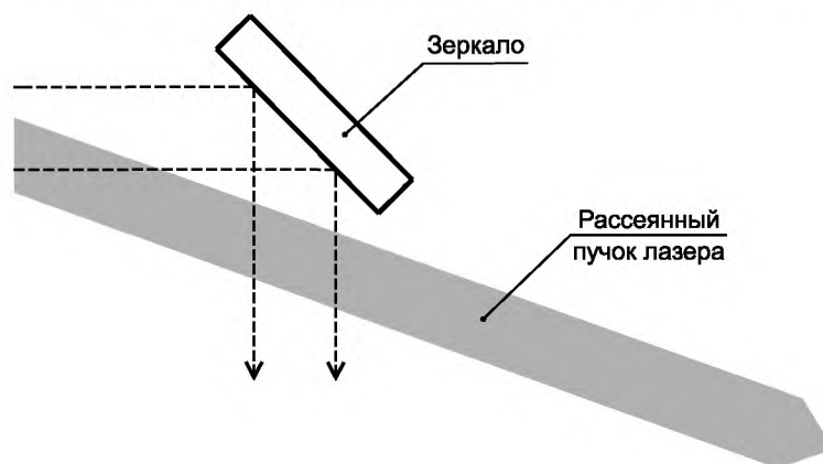
Рисунок В.4б — Отклонение луча от зеркала во время процедуры регулировки
