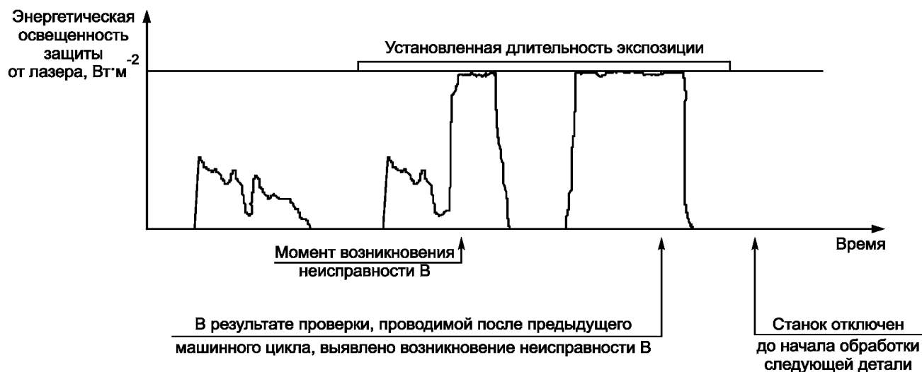
Рисунок В.6б — Отключение лазера при использовании автономного машинного мониторинга безопасности
