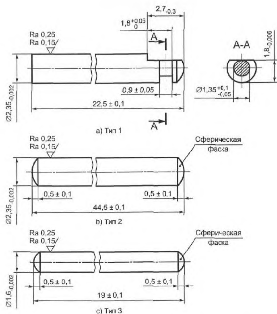
Рисунок 2 – Контрольные оправки
