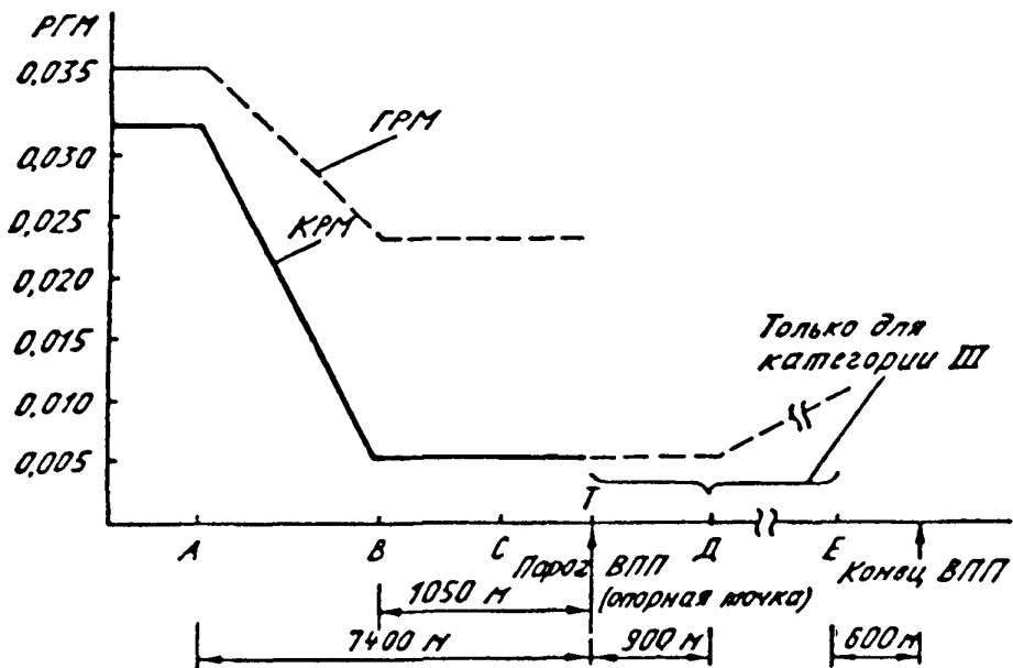
Рис. 2.4. Допустимые амплитуды искривлений линий курса и глассад для КРМ и ГРМ ИЛС II и III категорий.
