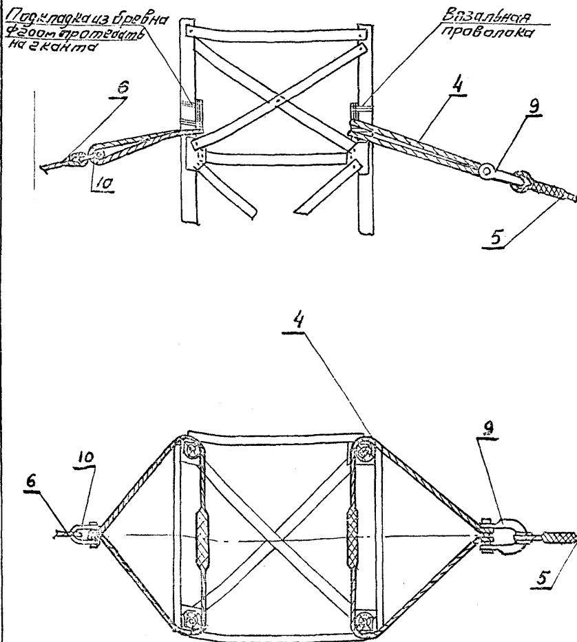
Рис. 5. Узел строповки слопы У110-1
