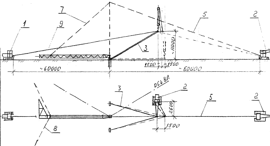
Рис. 9-2. Схема подъема латочной стрелы Н=22м
