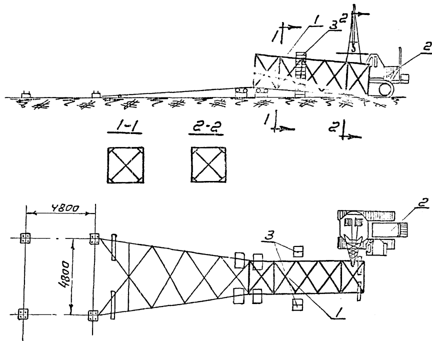
Рис. 5 Сборка 2-й секции ствoла опоры У110-1
