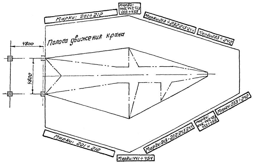
Рис. 2 Раскладка пакетов с деталями опоры У110-1 на пакете
