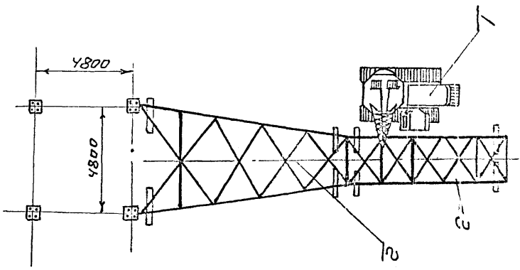
Рис. 4 Сборка нижней плоскости 1 й и 2 й секций ствoла
