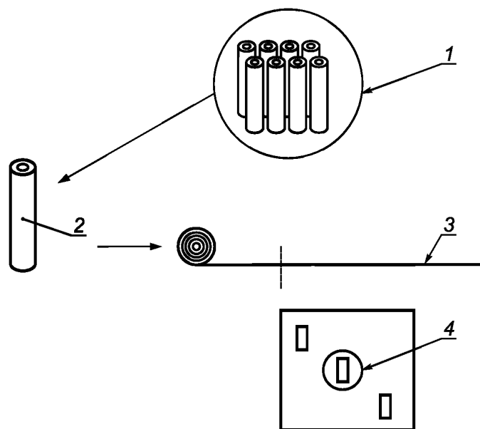
1 — партия; 2 — выборка; 3 — полоса материала; 4 — образцы для испытаний
