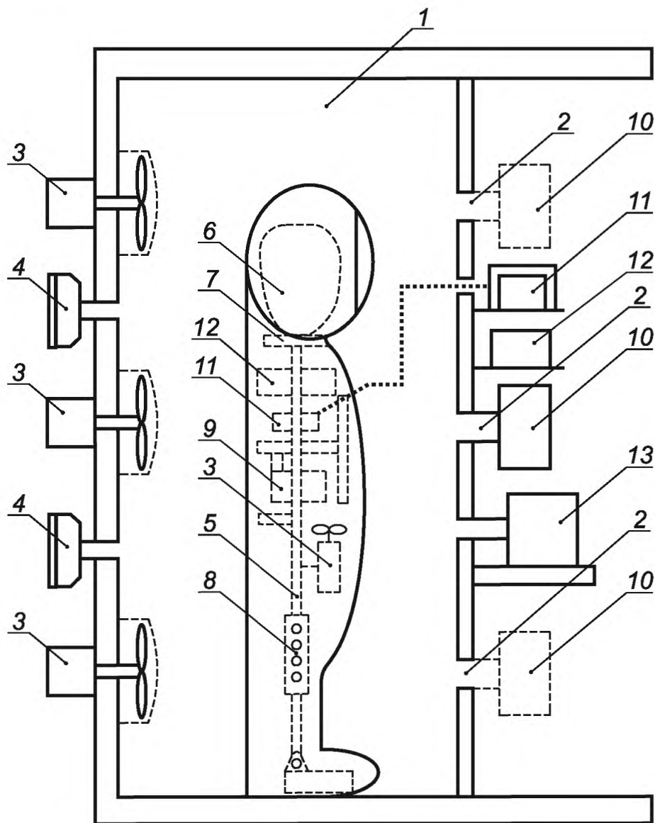
1 — герметичная испытательная камера; 2 — штуцер для отбора проб воздуха; 3 — электроклапан; 4 — противогазовая коробка; 5 — трубчатый манекен; 6 — муляж головы человека; 7 — плечевой каркас; 8 — регулятор высоты; 9 — устройство для имитации перепадов давлений; 10 — газоанализатор модельного газа в камере; 11 — газоанализатор модельного газа в подкостюмном пространстве; 12 — измеритель величин перепадов давлений; 13 — генератор модельного газа
